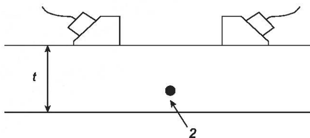
б) Контроль дифракционно-временным методом TOFD
