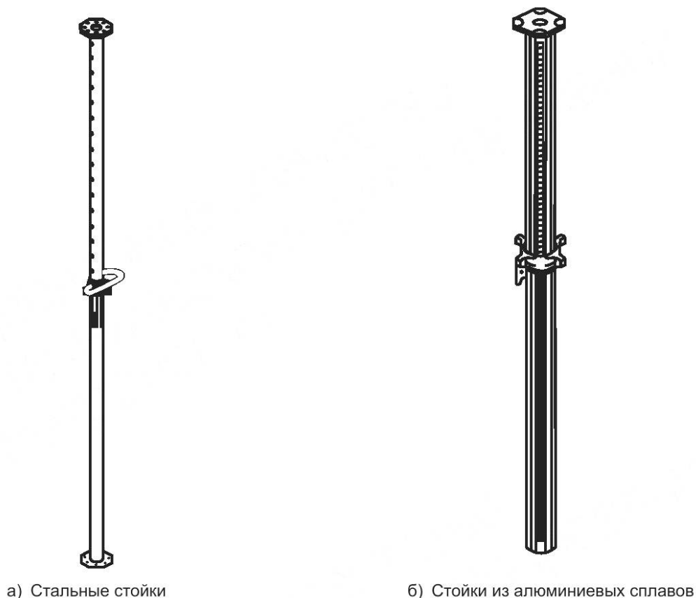
Рисунок 2 — Стойки для опалубки перекрытия
