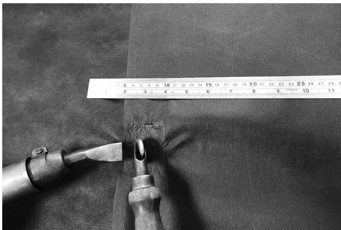
б — сварка нагретым газом с помощью строительного фена и прижимного ролика
