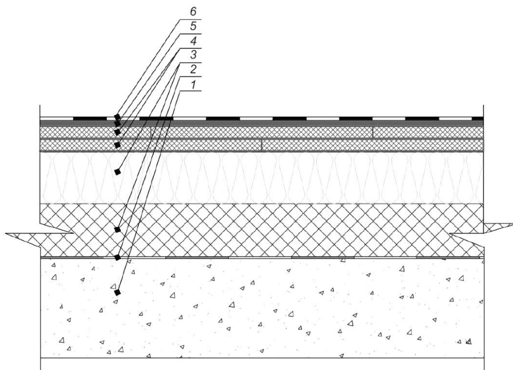
1 — основание (цементная стяжка, бетонная плита и т. п.); 2 — пароизоляция; 3 — теплоизоляция; 4 — уклонообразующий материал; 5 — слой; 6 — покрытие
