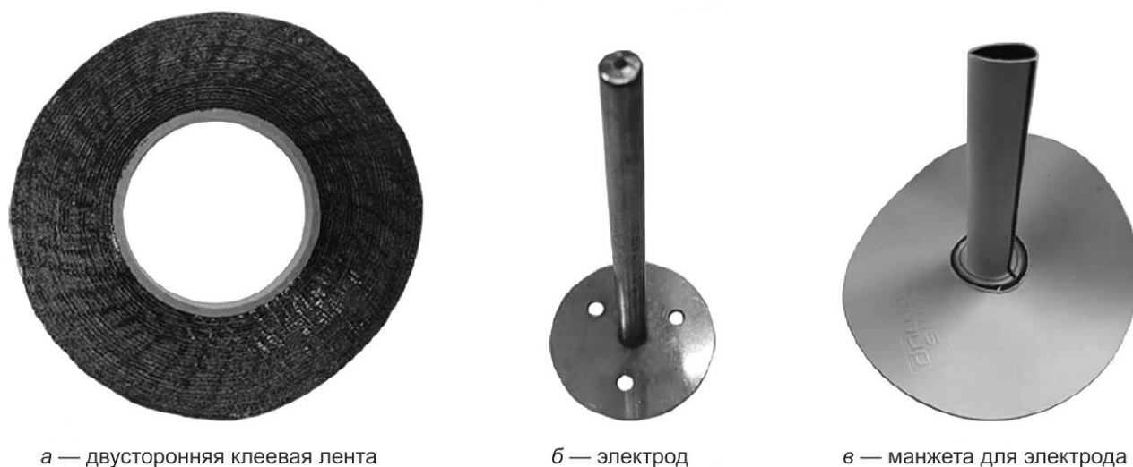
Рисунок 3 — Вспомогательные материалы для монтажа слоя
