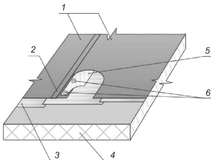
1 — покрытие; 2 — шов (клеевой, сварной); 3 — слой; 4 — основание крыши или подземной части здания/сооружения по проекту; 5 — лента из электропроводящего рулонного материала; 6 — механическое крепление покрытия
