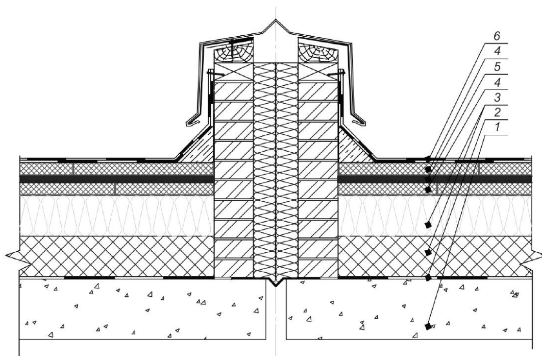
Рисунок В.3 — Схема монтажа слоя вблизи поперечного деформационного шва
