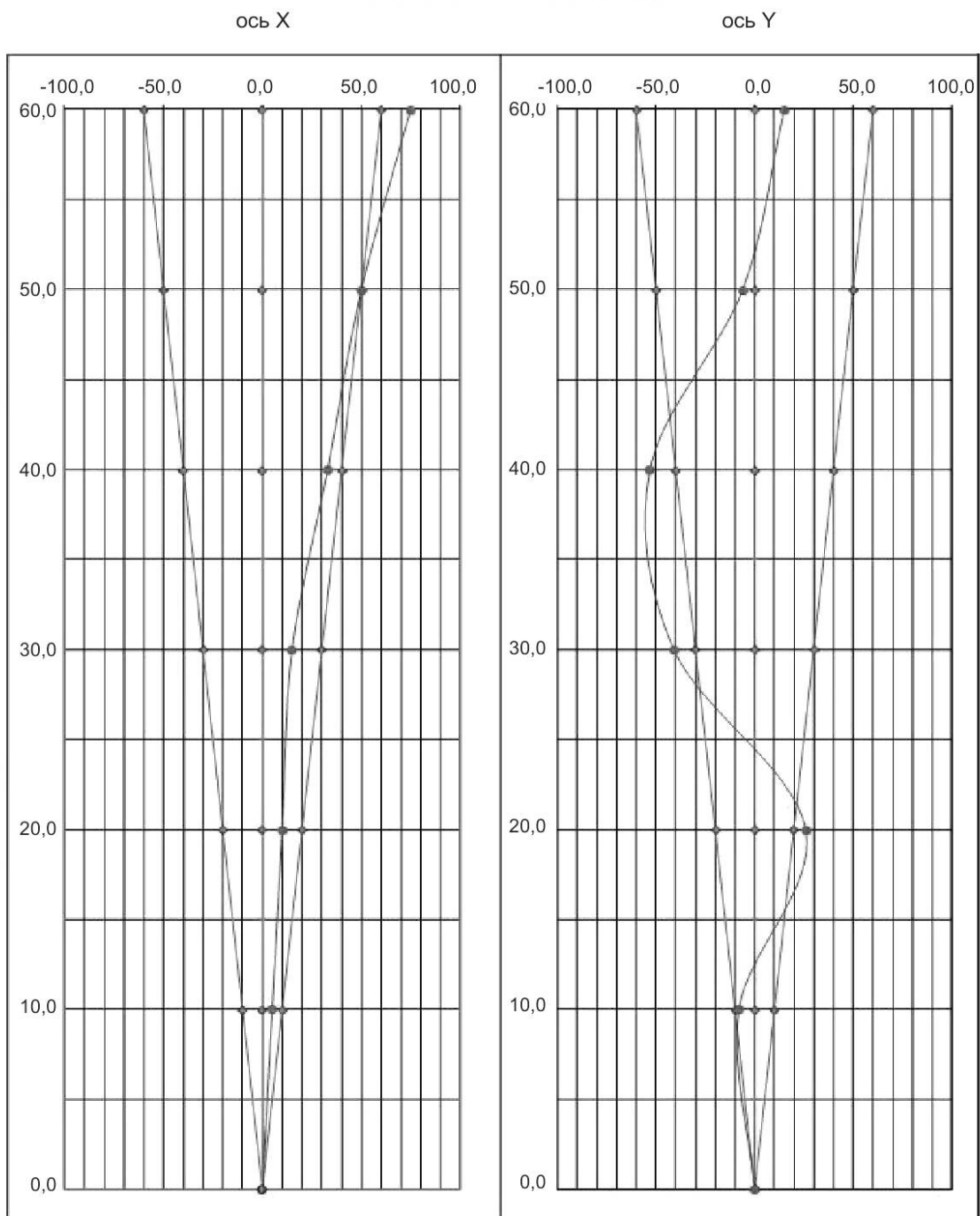
Рисунок Л.5 — Пример исполнительной схемы вертикальности оси ствола АО (две стоянки)
