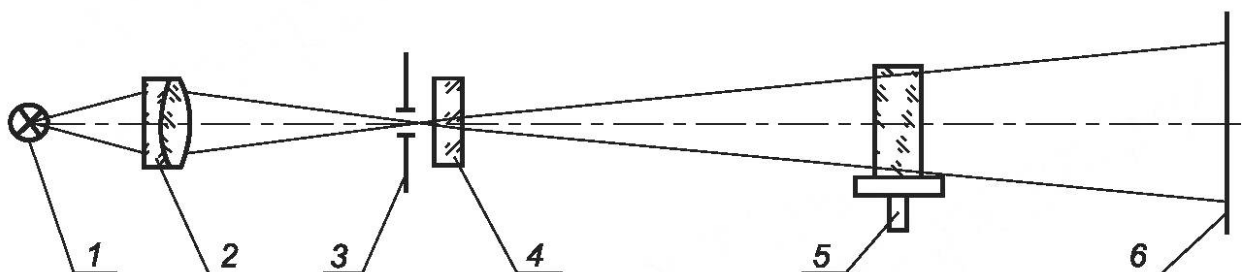
1 — источник излучения; 2 — конденсор; 3 — сменная диафрагма; 4 — светофильтр (или комплект светофильтров); 5 — держатель с испытуемым стеклом; 6 — экран
