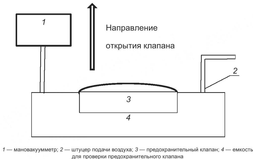
Рисунок 1 — Схема проверки работоспособности и регулировки предохранительного клапана с помощью емкости
