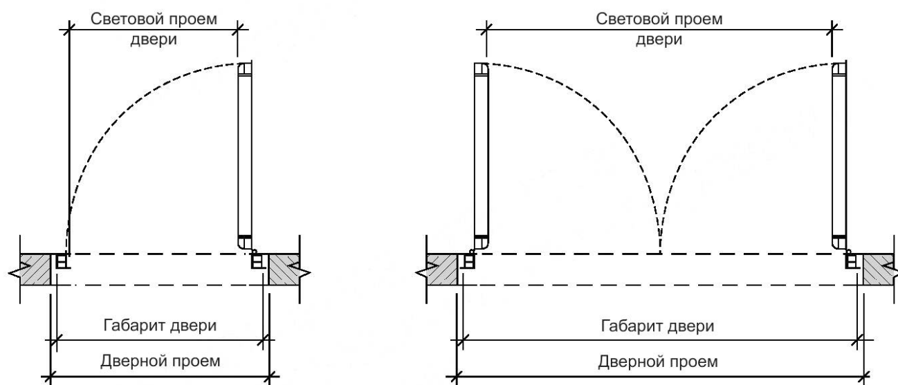
Рисунок 2 — Определение светового проема двери
