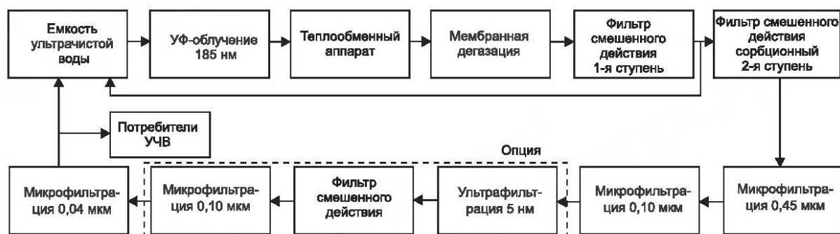
Рисунок Г.1 — Блок-схема участка получения УЧВ типов Е1.3, Е1.4 и ее распределение
