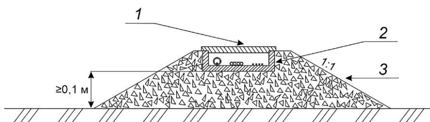
а) Лоток на специальной насыпи из щебня
