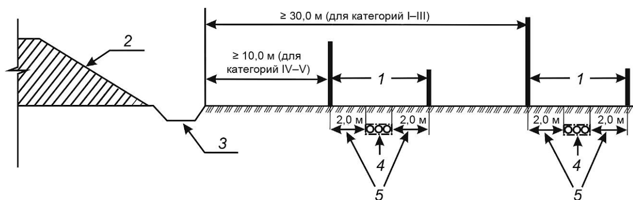
1 — граница охранной зоны ЛС; 2 — откос насыпи автомобильной дороги; 3 — водоотводная канава; 4 — ЛС; 5 — охранный зона ЛС
