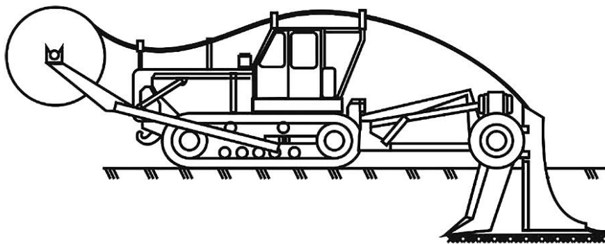
Рисунок 3 — Устройство ЛС методом пропорки
