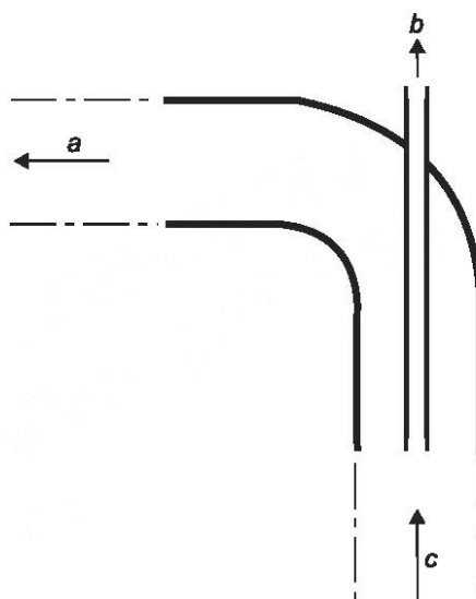
a — направление потока к побудителю расхода; b — направление потока к счетчику частиц, q_{pc} ; c — направление исходного потока, q_s
