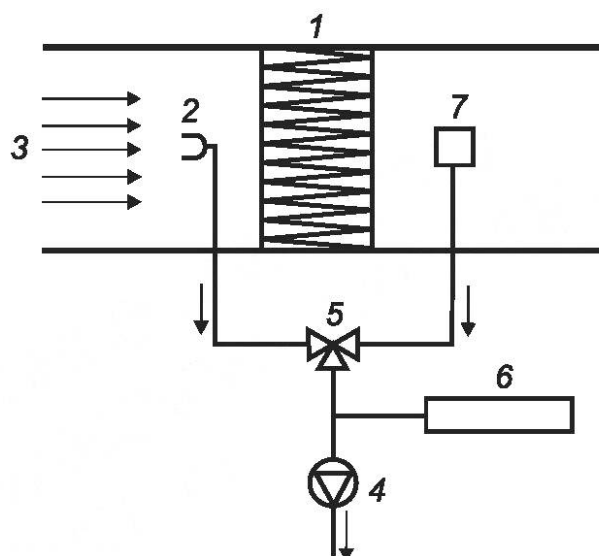
1 — испытательное устройство; 2 — воздушозаборное устройство до испытательного устройства; 3 — поток воздуха; 4 — побудитель расхода; 5 — клапан; 6 — счетчик частиц; 7 — НЕРА-фильтр после испытательного устройства
