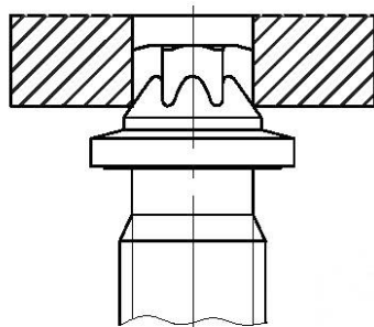
в) Проверка калибром В
