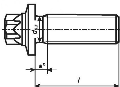
в) Винты с резьбой до головки (длины выше ступенчатой линии в таблице 2)
