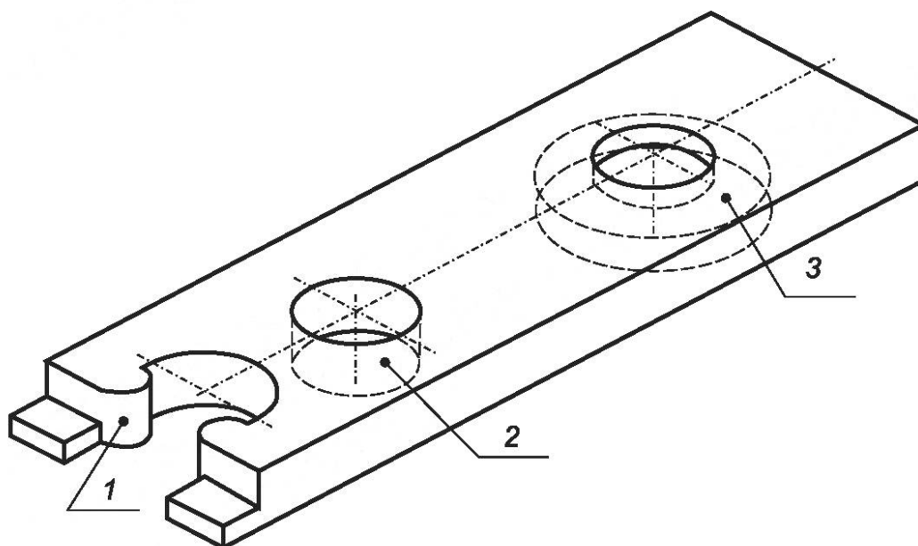
1 — калибр А; 2 — калибр В; 3 — калибр С
