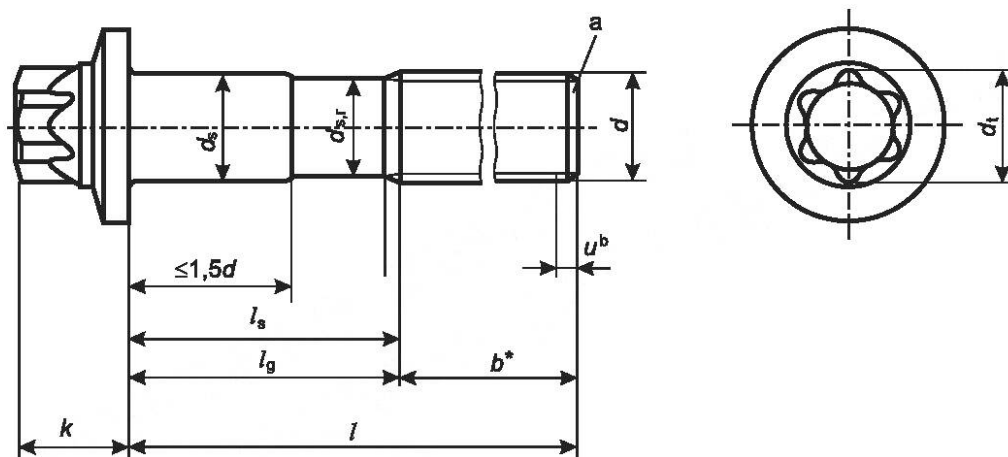
а) Винты с номинальной длиной l \geq 10d
