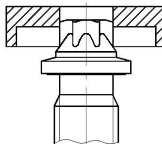
г) Проверка калибром С
