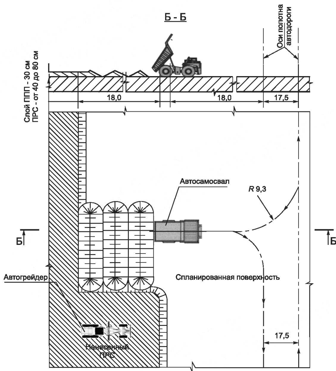
Рисунок Б.1 — Технологическая схема нанесения ПРС на поверхность отвала
