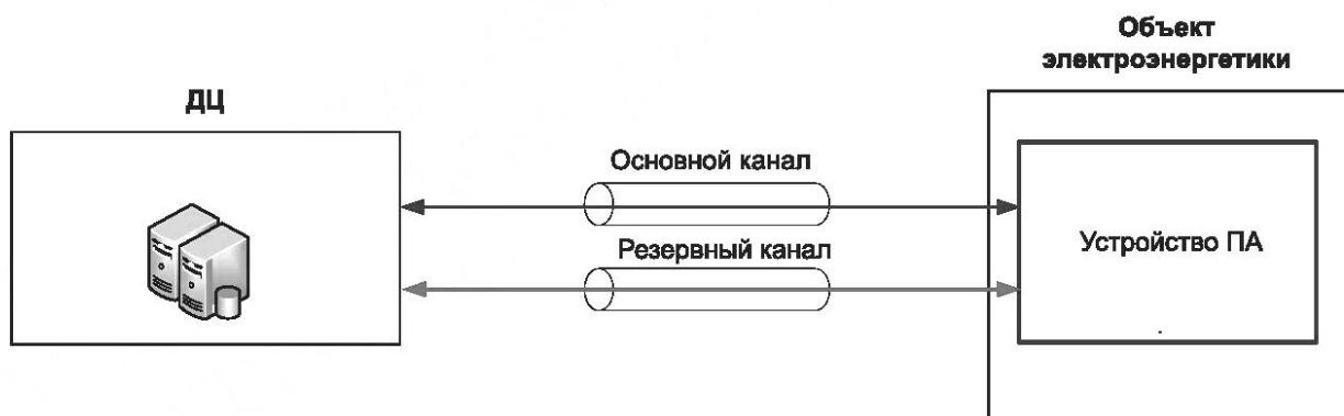
Рисунок А.1 — Вариант 1 — передача доаварийной телеметрической информации из ДЦ в установленное на объекте электроэнергетики устройство ПА с установкой прямого соединения на уровне протокола обмена
