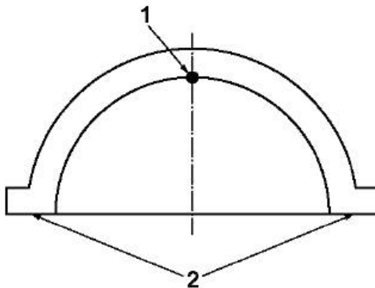
Рисунок А.1 — Расположение точек на сферической головке
