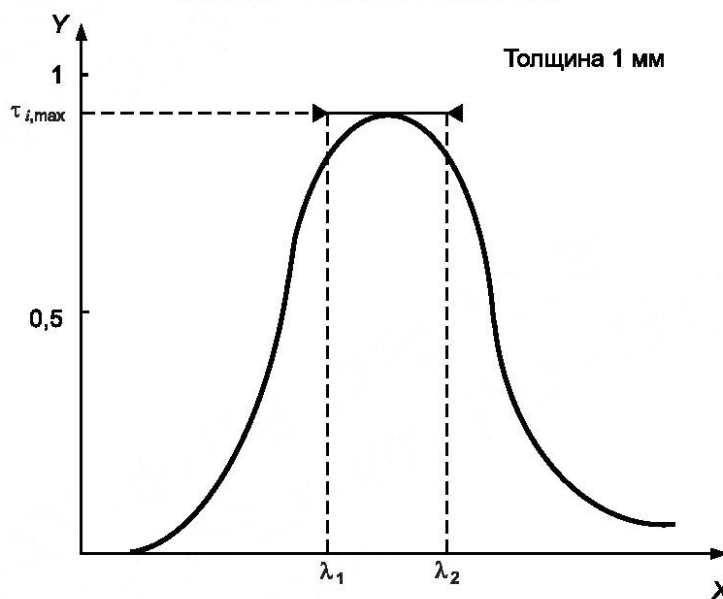
Рисунок 3 — Графическое представление спектральной характеристики полосового фильтра BP (указание диапазонов длин волн)
