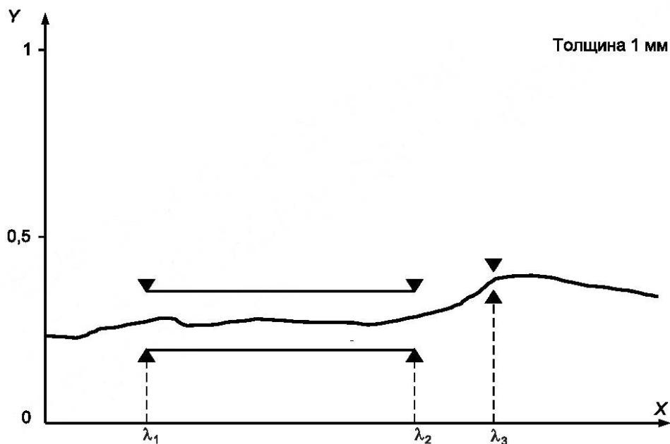
Рисунок 2 — Графическое представление спектральной характеристики ослабляющего фильтра ND
