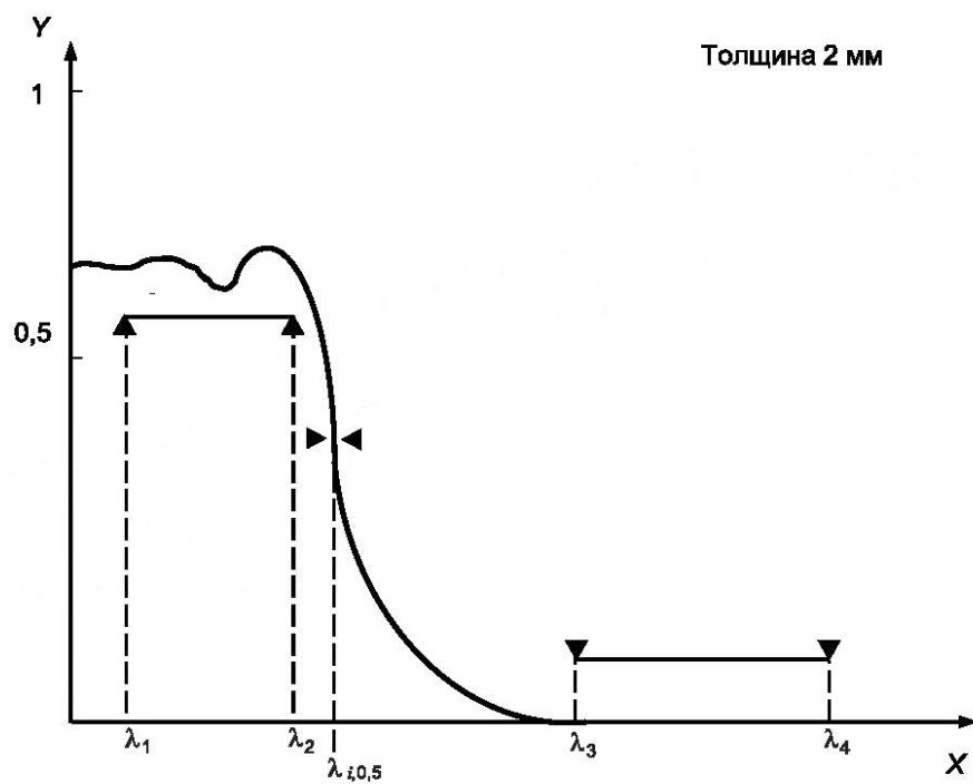
Рисунок 6 — Графическое представление спектральной характеристики коротковолново-пропускающего фильтра SP
