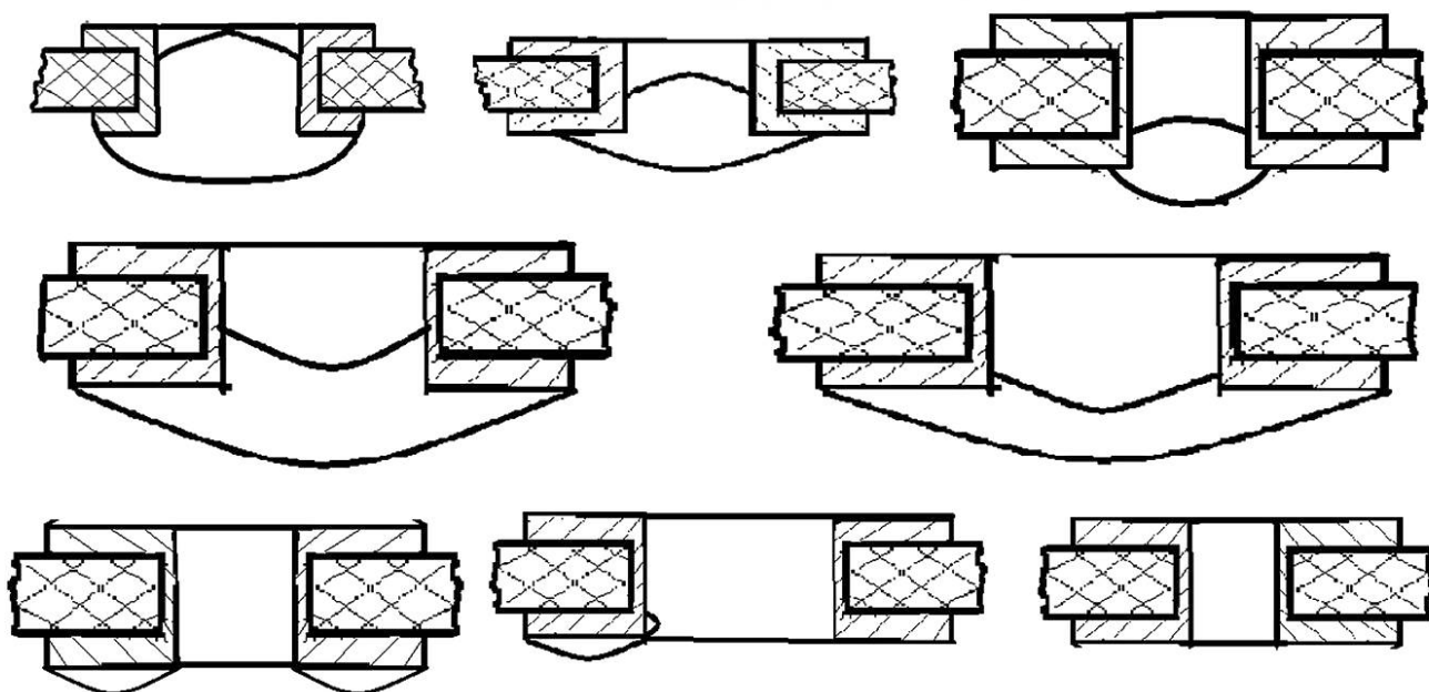
б — плохая паяемость отверстий
