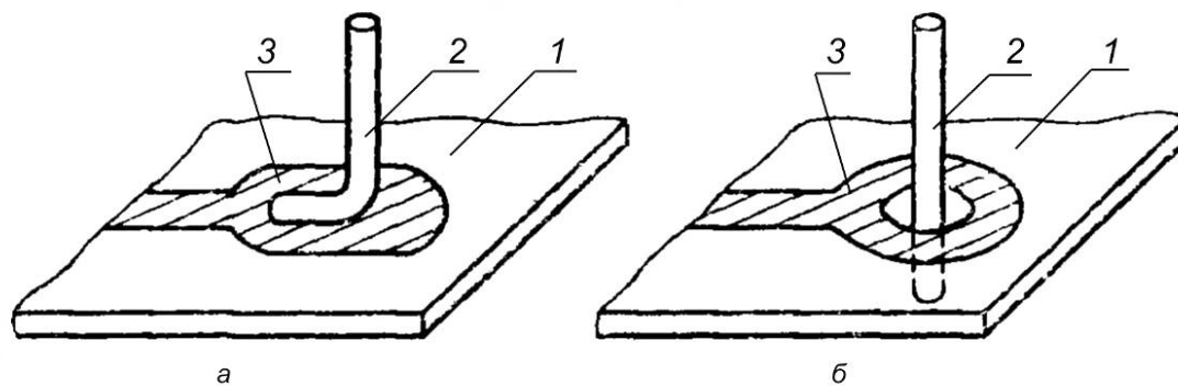
1 — плата; 2 — проволока; 3 — КП (металлизированное отверстие)
