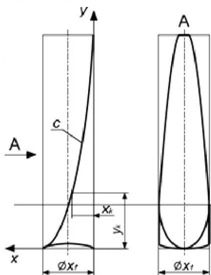
Рисунок 6 — Стабилизатор зонда щелевого типа
