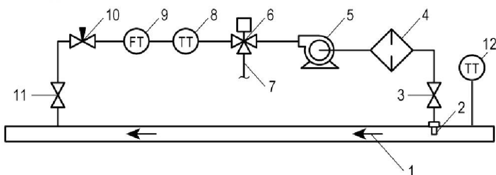
1 — направление потока; 2 — пробоотборный зонд; 3, 11 — вентили; 4 — фильтр; 5 — циркуляционный насос; 6 — трехходовой клапан; 7 — место подключения пробоотборника; 8, 12 — СИ температуры; 9 — СИ или индикатор расхода; 10 — регулятор расхода
