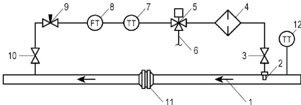
1 — направление потока; 2 — пробоотборный зонд; 3, 10 — вентили; 4 — фильтр; 5 — трехходовой клапан; 6 — место подключения пробоотборника; 7, 12 — СИ температуры; 8 — СИ или индикатор расхода; 9 — регулятор расхода; 11 — сужающее устройство
