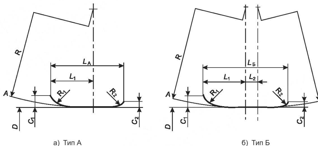
Рисунок 1 — Типы профилей А и Б
