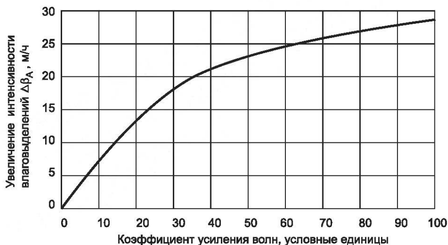
Рисунок 2 — Влияние воздействия водных аттракционов на увеличение интенсивности влаговывделений
