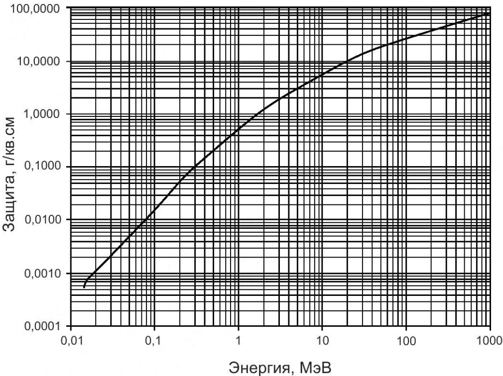
Рисунок Б.1 — Зависимость энергии проникновения электронов от эквивалентной защиты конструкцией АКА
