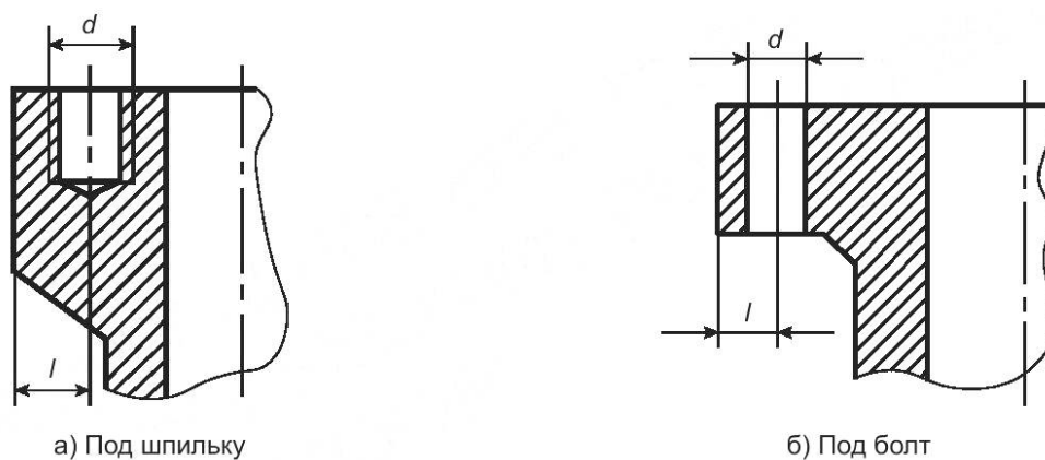
Рисунок 4.5 — Расположение отверстий
