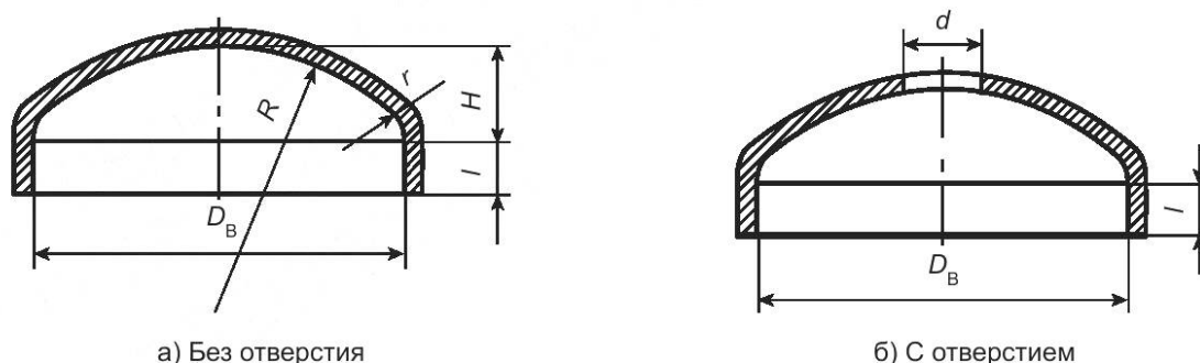
Рисунок 4.2 — Торосферическое днище
