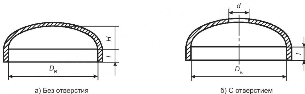
Рисунок 4.1 — Эллиптическое днище
