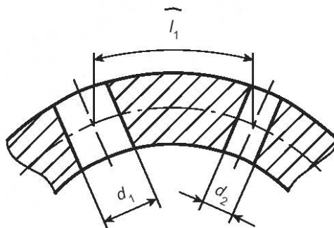
Рисунок 4.3 — Расположение отверстий на криволинейной поверхности
