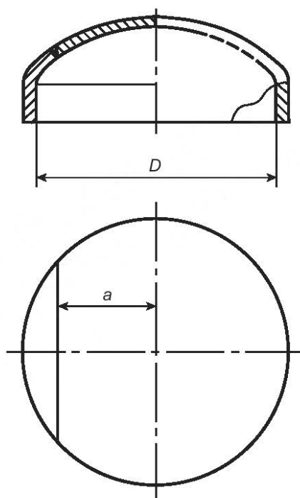
Рисунок 4.8 — Расположение хордовых швов
