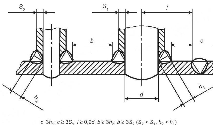
Рисунок 4.10 — Расположение сварных соединений приварки патрубков
