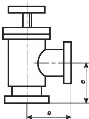
Рисунок 1 — Угловой клапан
