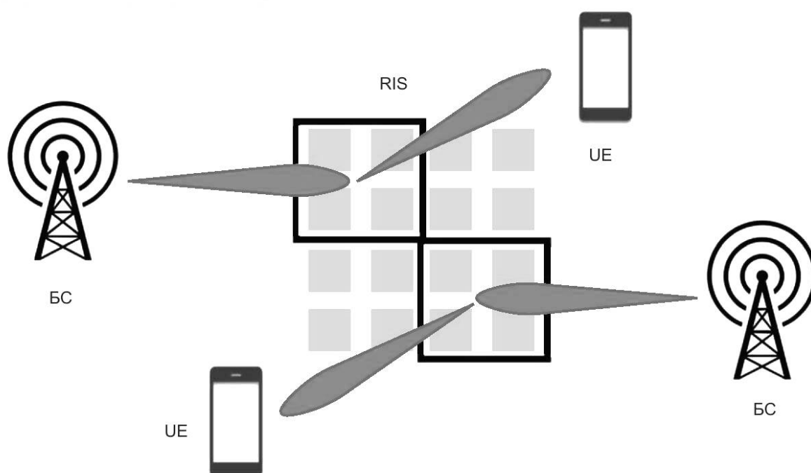
Рисунок 10 — Пример множественного доступа к радиосети с RIS
