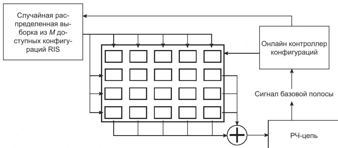
Рисунок 3 — Структурная схема аппаратной архитектуры RIS, включающая в себя одну активную РЧ-цепь приема, обеспечивающую обнаружение принимаемого сигнала в базовой полосе частот
