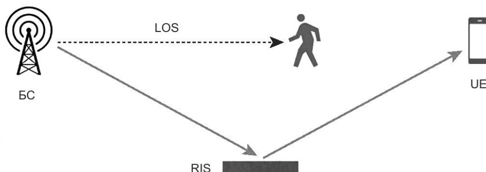
Рисунок 4 — Применение RIS для устранения блокировки LOS внутри и вне помещений
