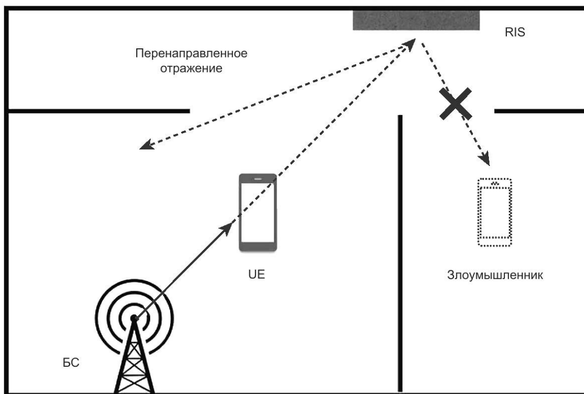
Рисунок 11 — Перенаправление RIS отраженных радиосигналов в конкретную заданную область
