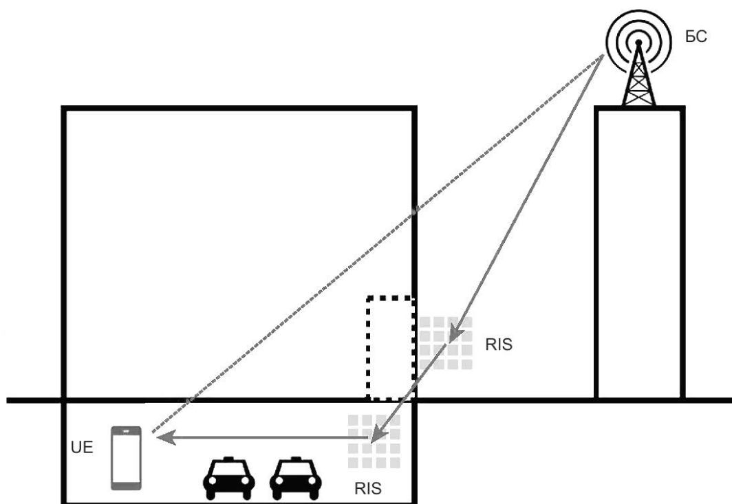
Рисунок 8 — Использование RIS для улучшения покрытия в сценарии, когда БС, расположенная на улице, обслуживает UE, которое находится в помещении
