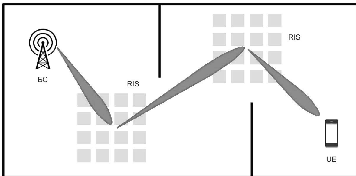
Рисунок 6 — Каскадное устранение блокировки LOS с помощью RIS
