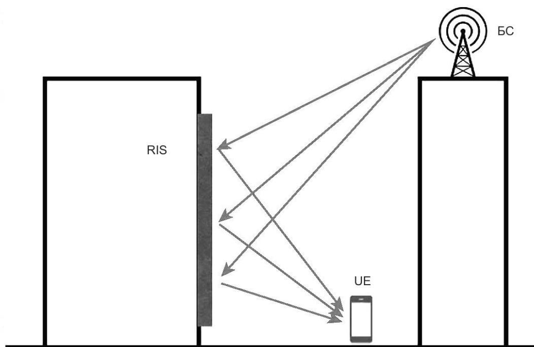
Рисунок 7 — Сценарий использования RIS вне помещения
