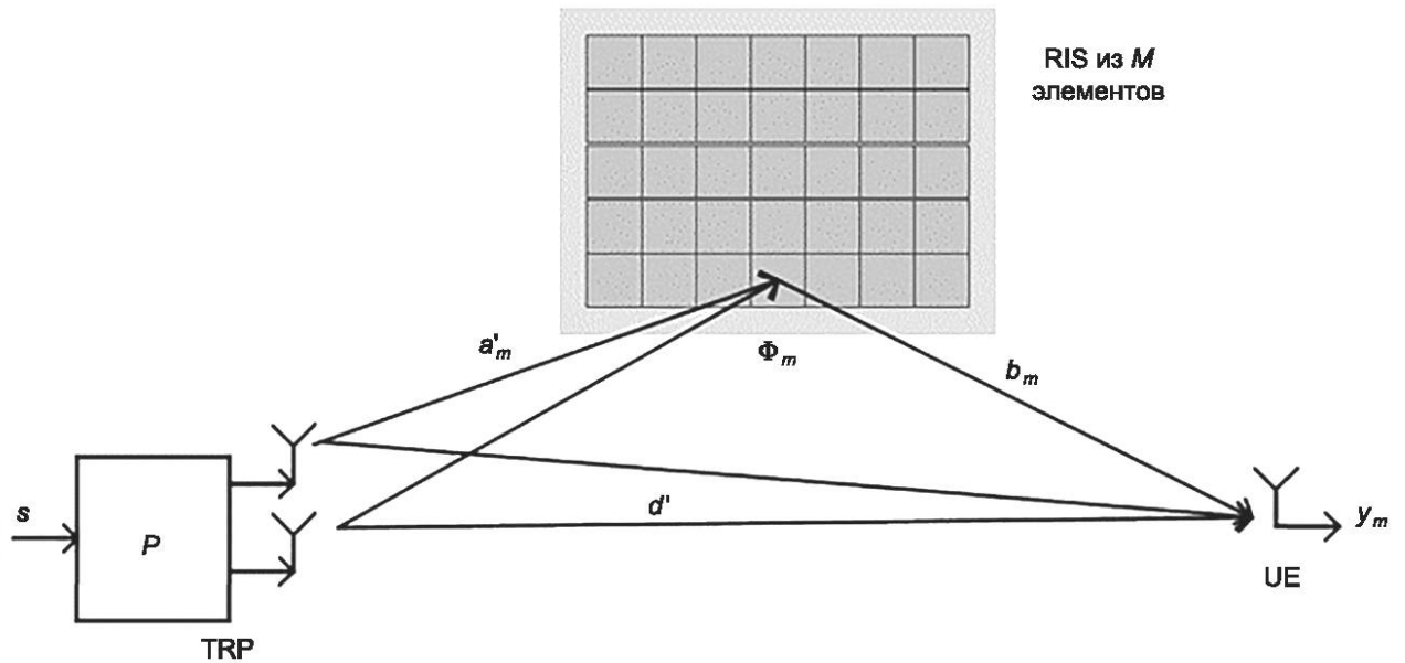
Рисунок 12 — Поэлементная оценка каналов с RIS в модели системы, включающей один элемент RIS
