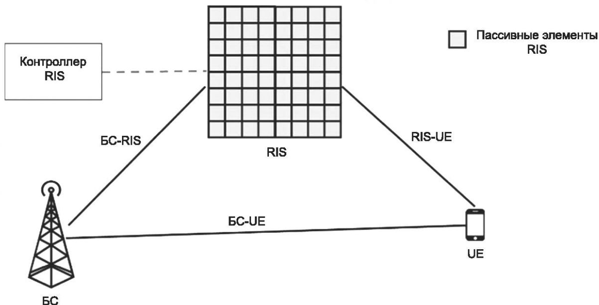
Рисунок 9 — Сценарий использования RIS, в котором RIS не выполняет встроенную оценку канала
