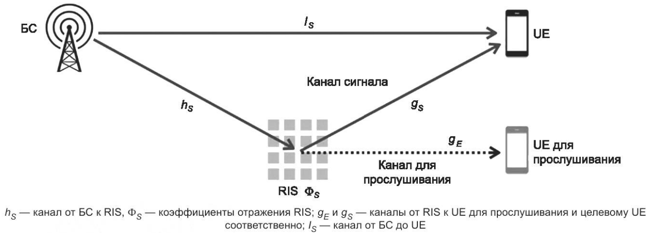
Рисунок 5 — Прослушивание сигнала от RIS
