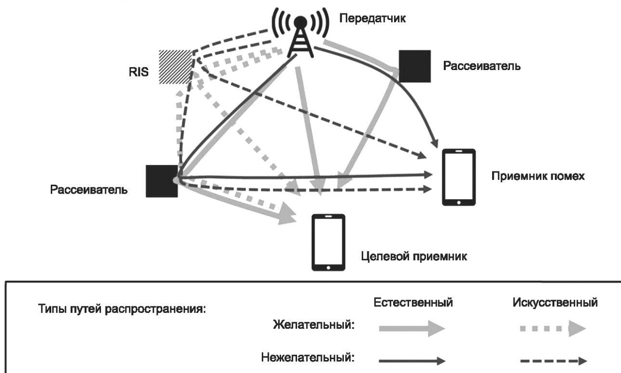
Рисунок 2 — Связь между передатчиком и целевым приемником, а также искусственные каналы распространения помех в беспроводной сети с RIS
