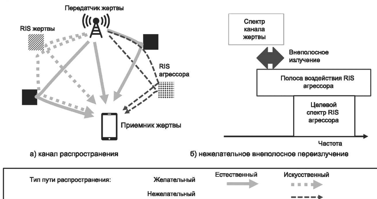
Рисунок 3 — Искусственные каналы распространения помех в беспроводных сетях связи, в которых использована RIS агрессора
