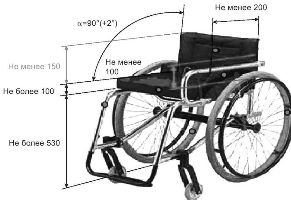
Рисунок 1 — Конструкция спортивной коляски для фехтования для спортсмена с правой фехтующей рукой
