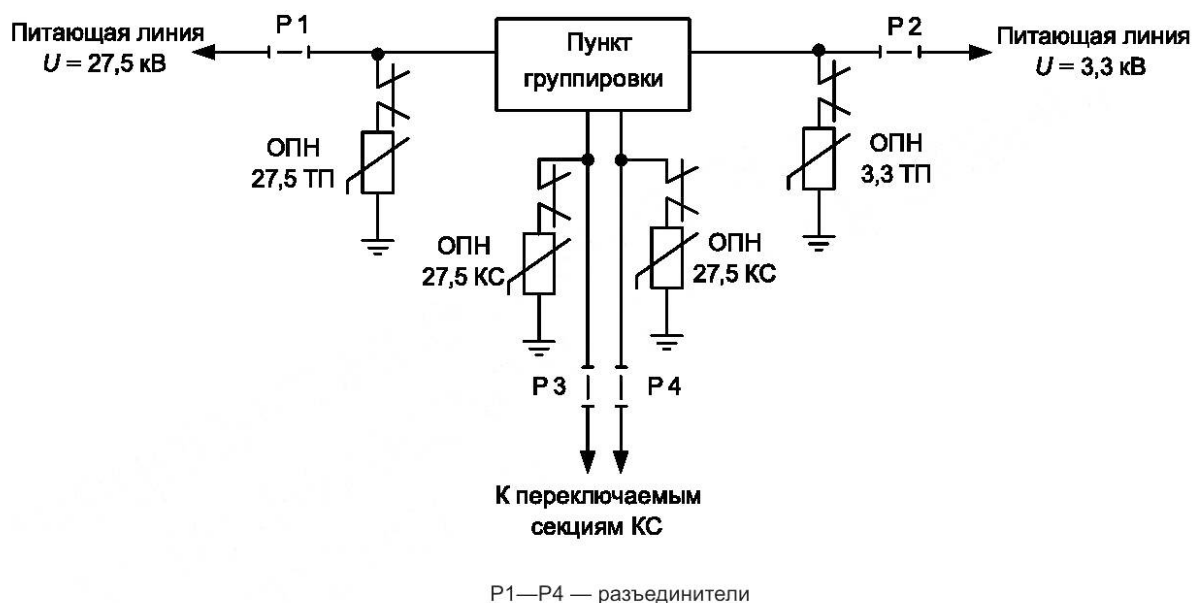
Рисунок 12 — Места установки ОПН на пункте группировки
