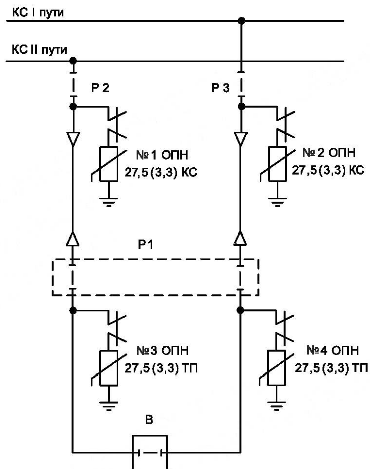
P1—P3 — разъединители; В — выключатель
