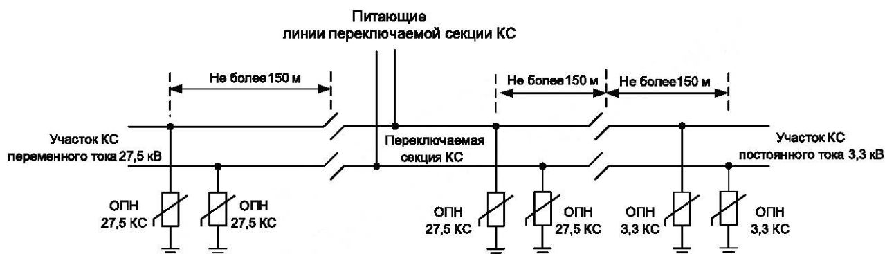
Рисунок 13 — Места установки ОПН на станции стыковки
