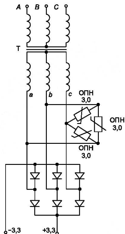
Рисунок 3 — Места установки ОПН на вентильных обмотках при применении схемы преобразования «трехфазная мостовая»
