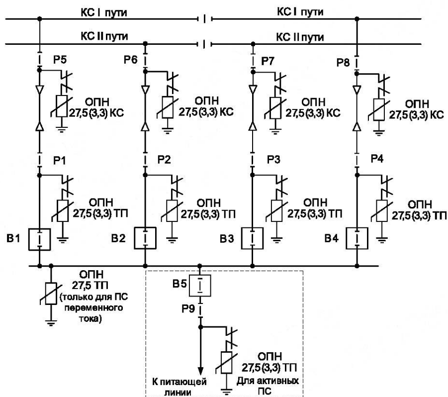
Рисунок 7 — Места установки ОПН на ППС с воздушным вводом для двухпутного участка
