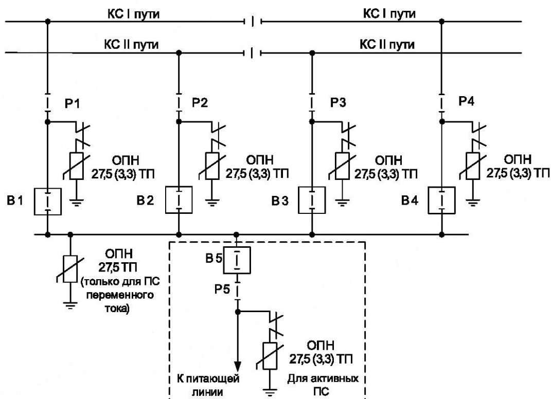
Рисунок 6 — Места установки ОПС на ПС с воздушным вводом для двухпутного участка
