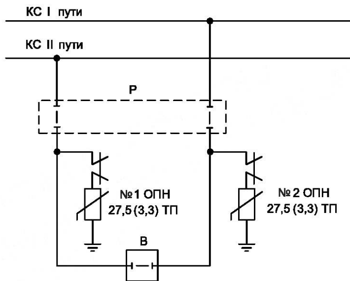
Рисунок 7 — Места установки ОПН на ППС с воздушным вводом для двухпутного участка
