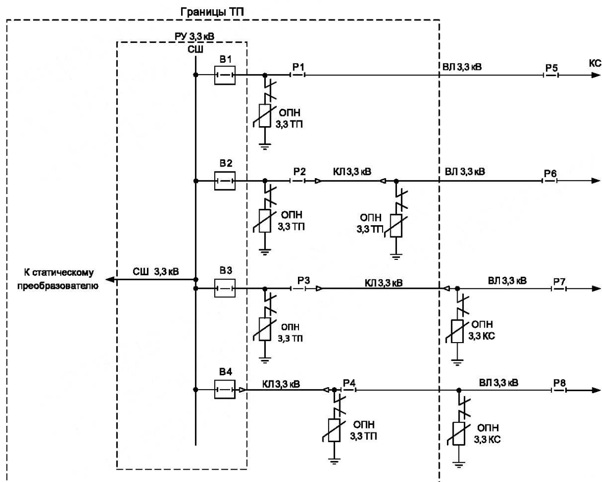
Рисунок 5 — Места установки ОПН в РУ и на питающих линиях на тяговой подстанции постоянного тока
