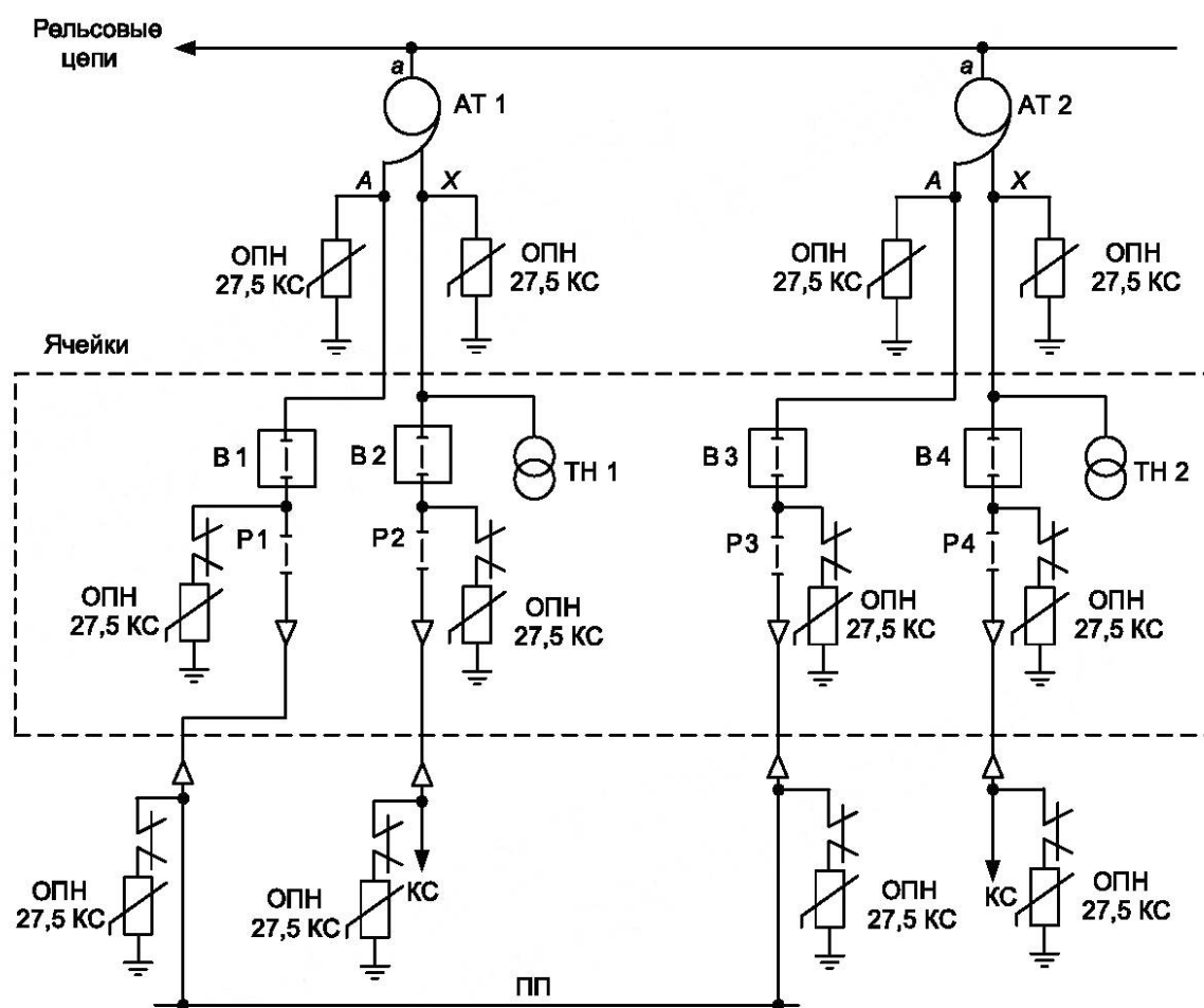
АТ 1, АТ 2 — автотрансформаторы; А, X, а — выводы автотрансформатора; ТН1, ТН2 — трансформаторы напряжения; В1—В4 — выключатели; Р1—Р4 — разъединители; ПП — питающий провод
