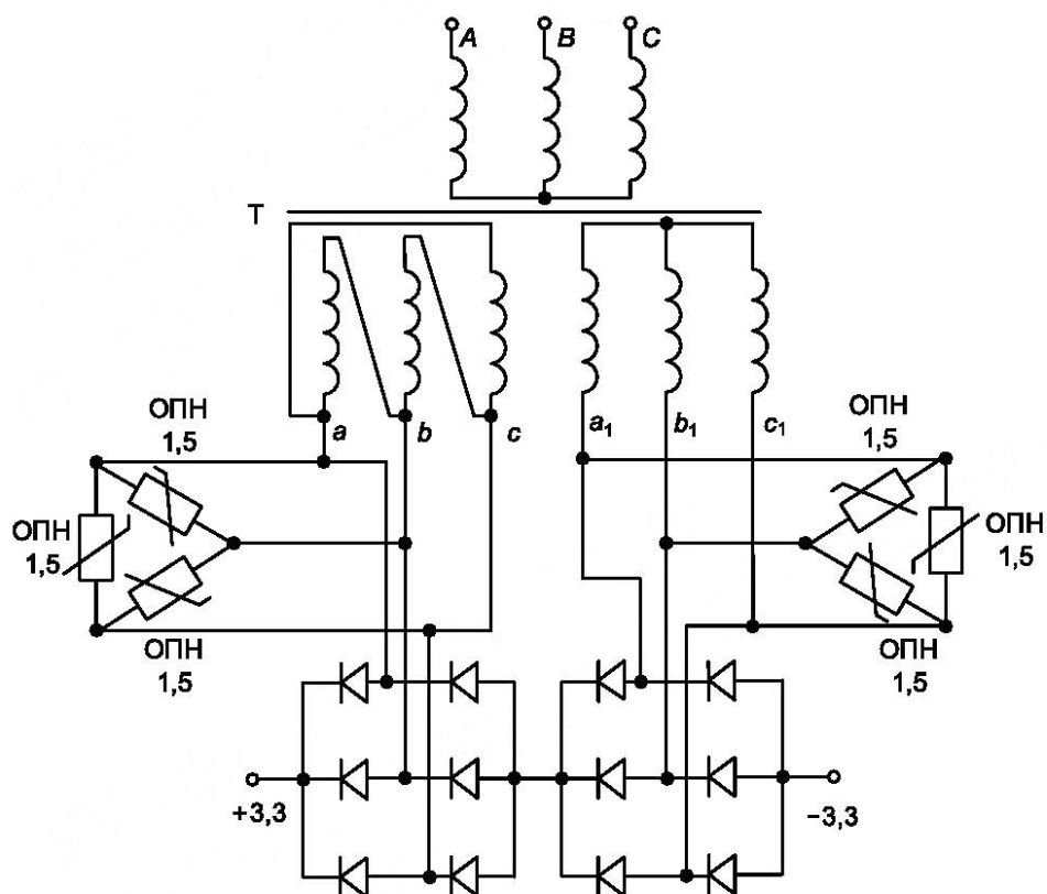
Рисунок 3 — Места установки ОПН на вентильных обмотках при применении схемы преобразования «трехфазная мостовая»
