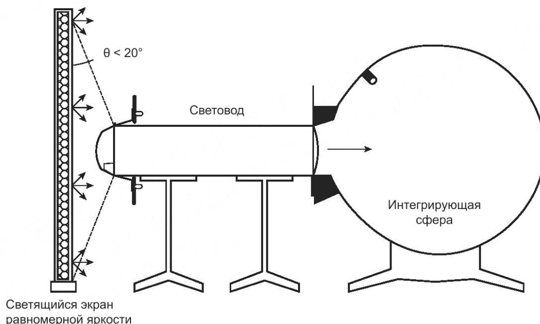
Рисунок 4.1 — Схема определения коэффициента пропускания компонентов световода
