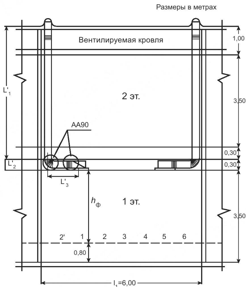
Рисунок Б.1 — Размещение трубчатых световодов естественного света на разрезе здания
