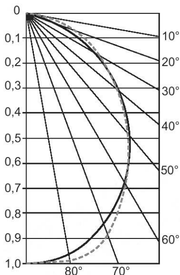
Рисунок Б.5 — Аппроксимация экспериментальной кривой функцией f(\alpha) = \cos^{1,7} \alpha
