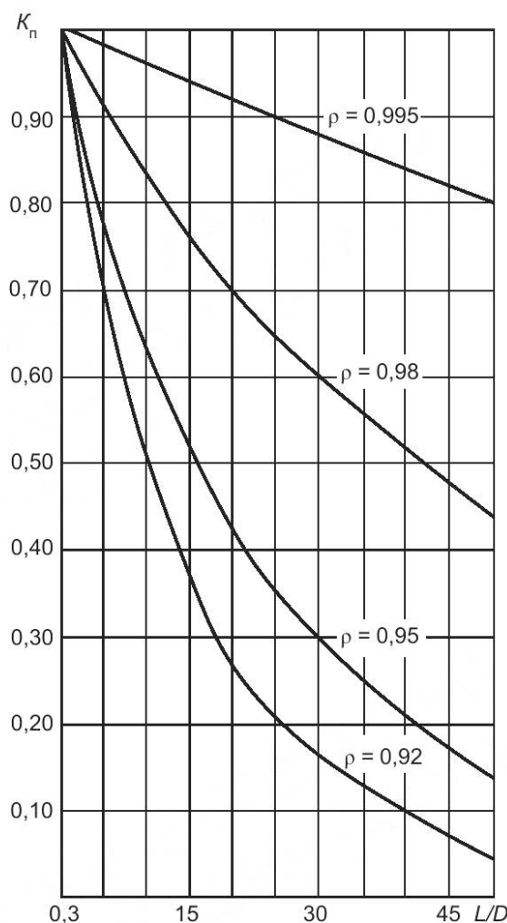
Рисунок 5.3 — График для определения коэффициента передачи светового потока K_n , зависящий от коэффициента отражения зеркального покрытия световодной трубы \rho и от отношения длины световода L к его диаметру D
