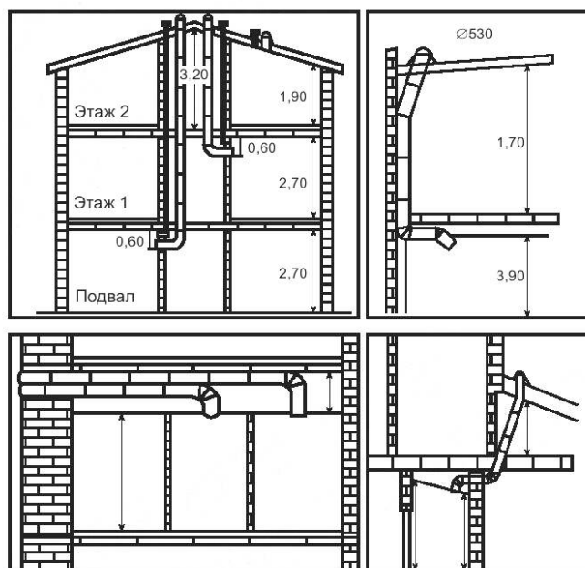
в) Возможные схемы размещения световодов
