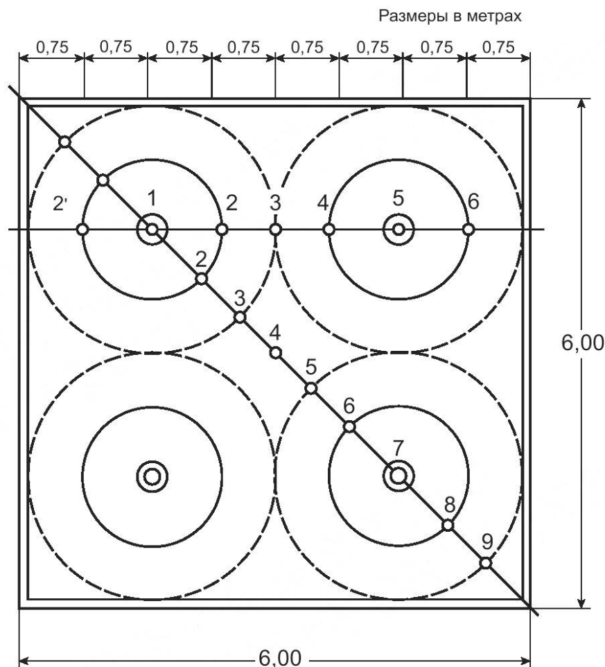
Рисунок Б.2 — Размещение трубчатых световодов естественного света на плане помещения (с изолиниями КЕО от каждого световода)
