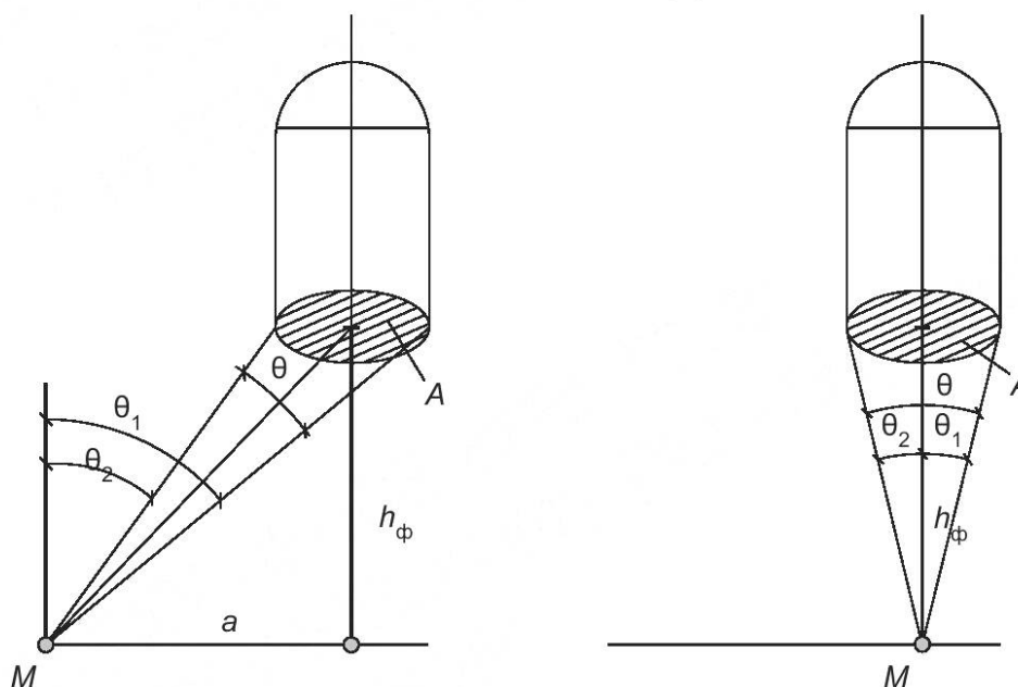
Рисунок 5.1 — К расчету коэффициента естественной освещенности от трубчатого световода
