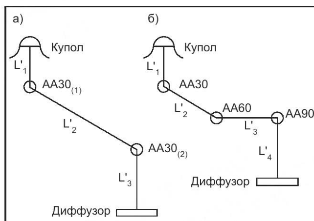
а) Схема световода с тремя коленами; б) Схема световода с четырьмя коленами
