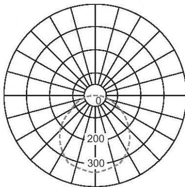
Рисунок Б.7 — Внешний вид, кривая силы света в полярных координатах световода естественного света диаметром 400 мм
