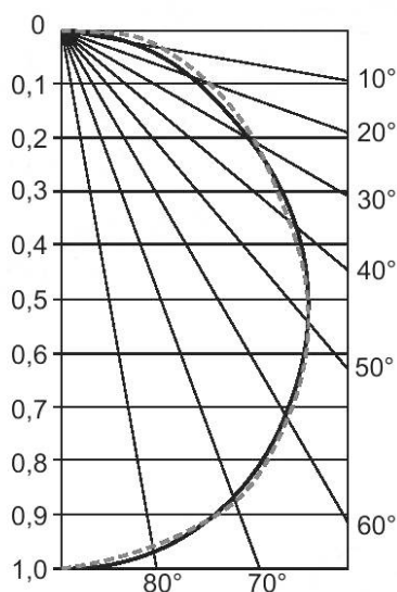
Рисунок Б.8 — Аппроксимация экспериментальной кривой функцией f(\alpha) = \cos^{1,3} \alpha
