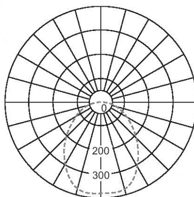
Рисунок Б.4 — Кривая силы света рассеивателя выходного отверстия световода диаметром 700 мм в полярных координатах
