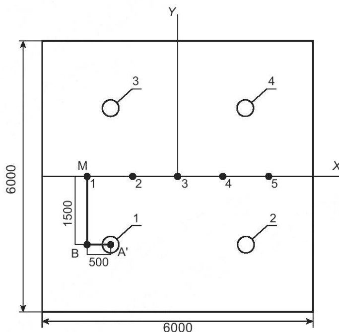
Рисунок Б.3 — Расположение световодов в помещении
