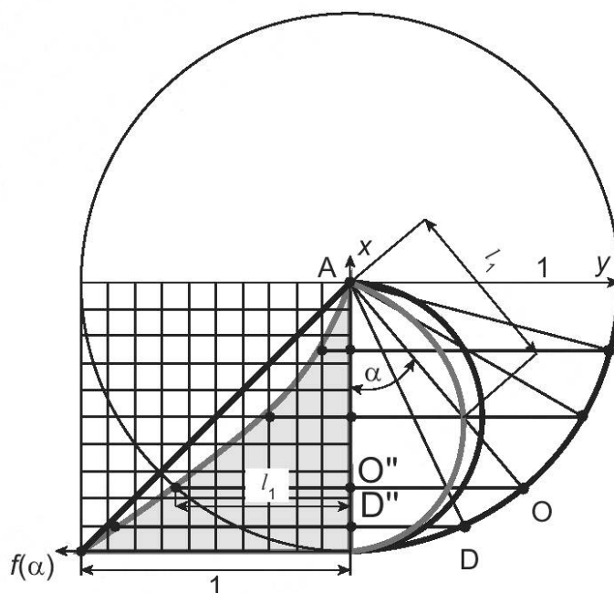
Рисунок 5.4 — Определение эквивалентного телесного угла при расчете светового потока по методу Руссо
