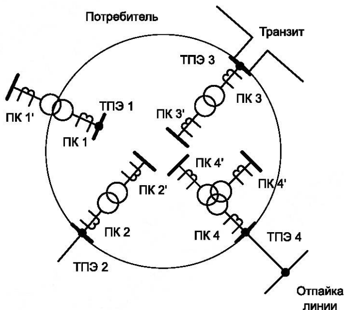
Рисунок Б.1 — Выбор пунктов контроля при различных способах присоединения потребителя (объекта генерации) к энергосистеме
