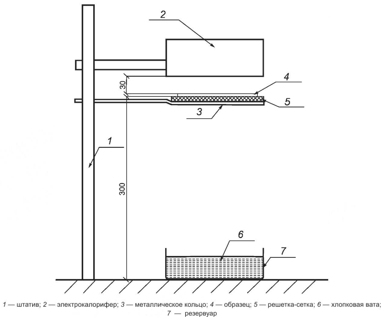
Рисунок В.2 — Схема установки для испытания образца для определения характеристик плавления (размеры приведены в миллиметрах)
