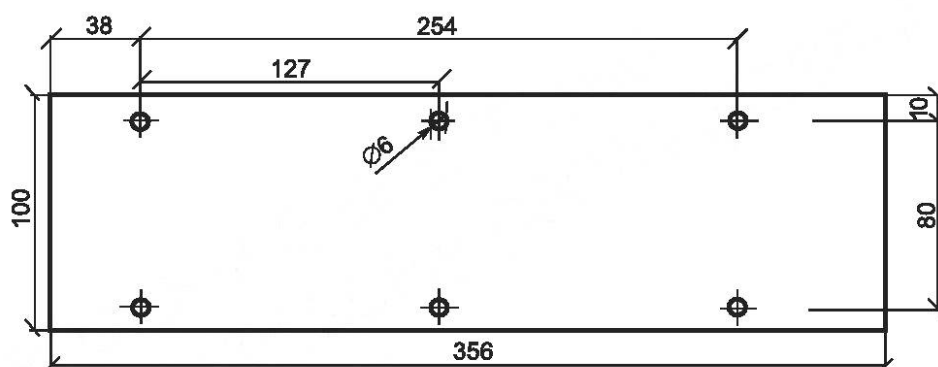
Рисунок А.1 — Образец материала (размеры в миллиметрах)
