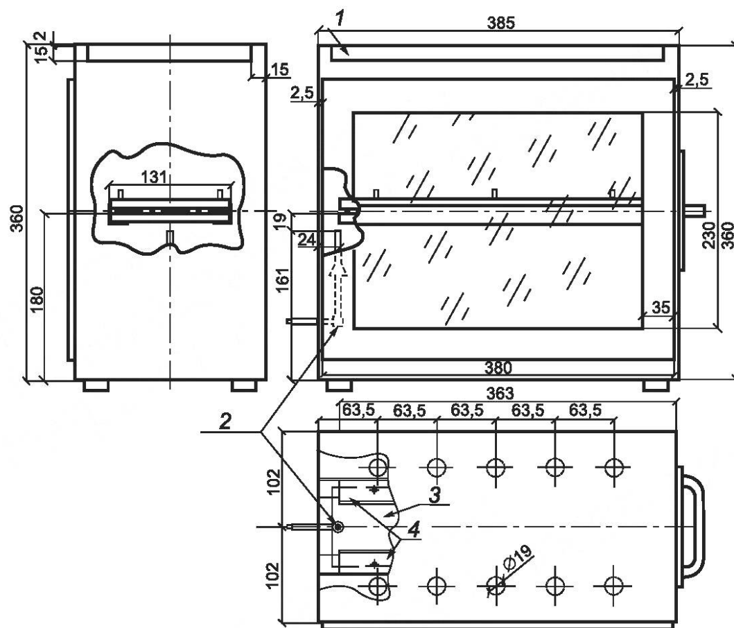
1 — вентиляционная прорезь; 2 — горелка Бунзена; 3 — поддон; 4 — держатель образца
