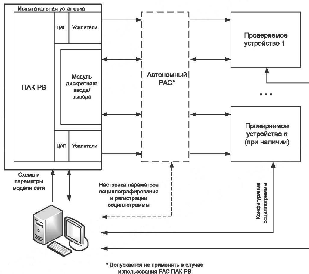
Рисунок А.4 — Структурная схема испытательной установки
