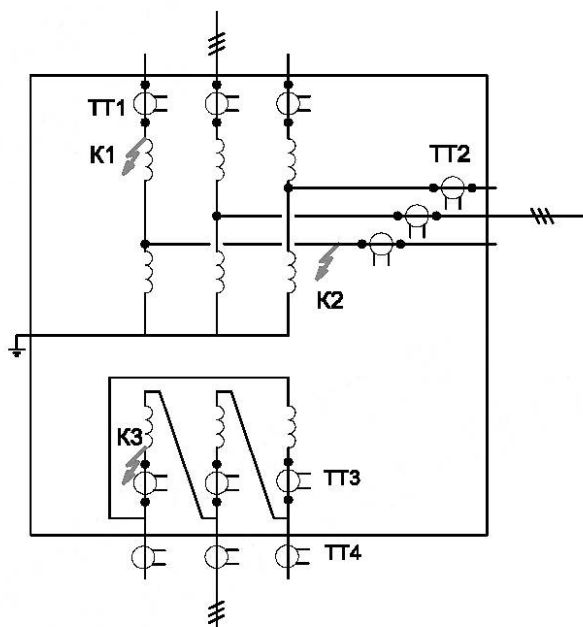
Рисунок А.2 — Уточнение расположения точек К3 внутри АТ
