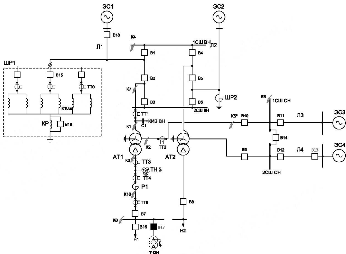
Рисунок А.1 — Тестовая модель энергосистемы для испытания устройств РЗА АТ (Т) 330 кВ и выше
