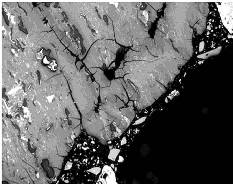
Рисунок А.11 — Краевые клиновидные трещины, разветвленные трещины, пустоты выщелачивания
