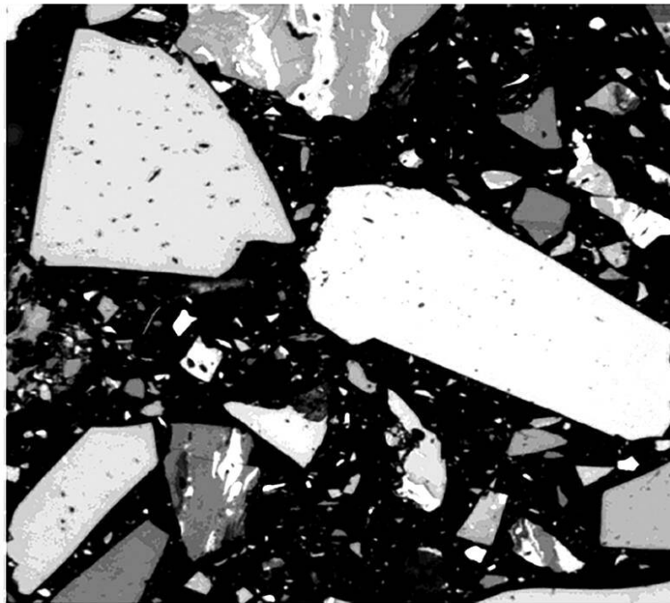
Рисунок А.1 — Неокисленные угольные зерна без признаков окисления
