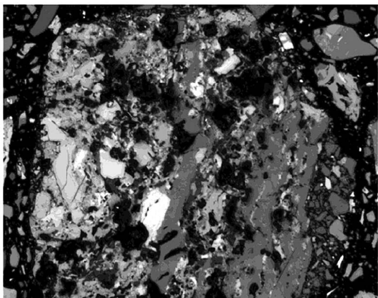
Рисунок А.14 — Дезинтеграция зерна угля с пустотами и кавернами
