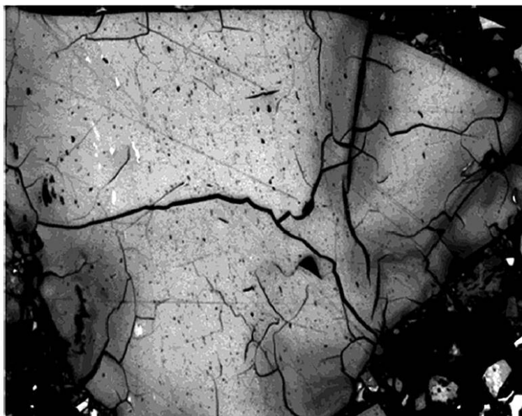
Рисунок А.9 — Клиновидные и разветвленные трещины, проникающие в глубину зерна, некоторые с понижением рельефа витринита
