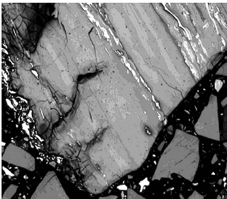
Рисунок А.4 — Клиновидные трещины и глубокие трещины с понижением рельефа и изменением цвета витринита по краям трещин
