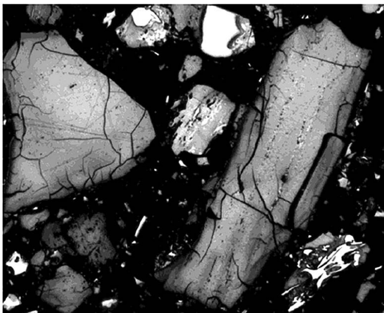
Рисунок А.7 — Клиновидные и разветвленные трещины
