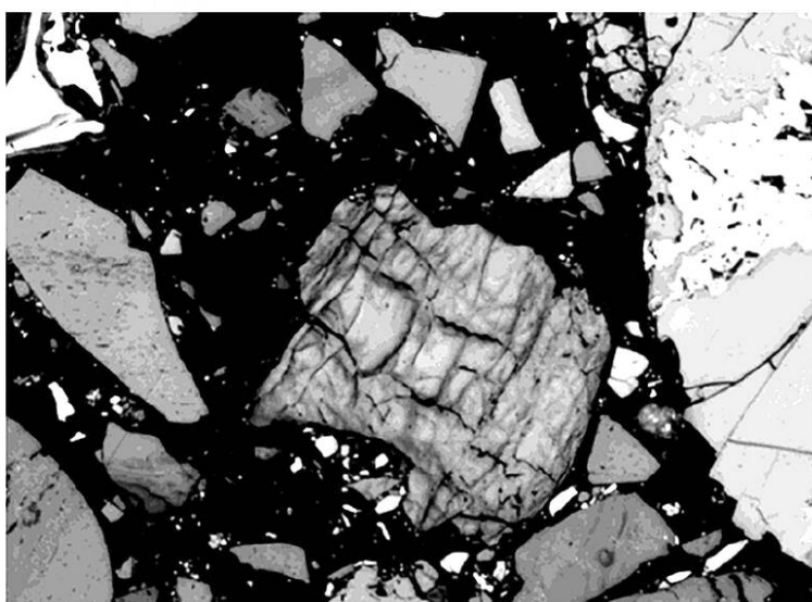
Рисунок А.12 — Дезинтеграция частицы угля
