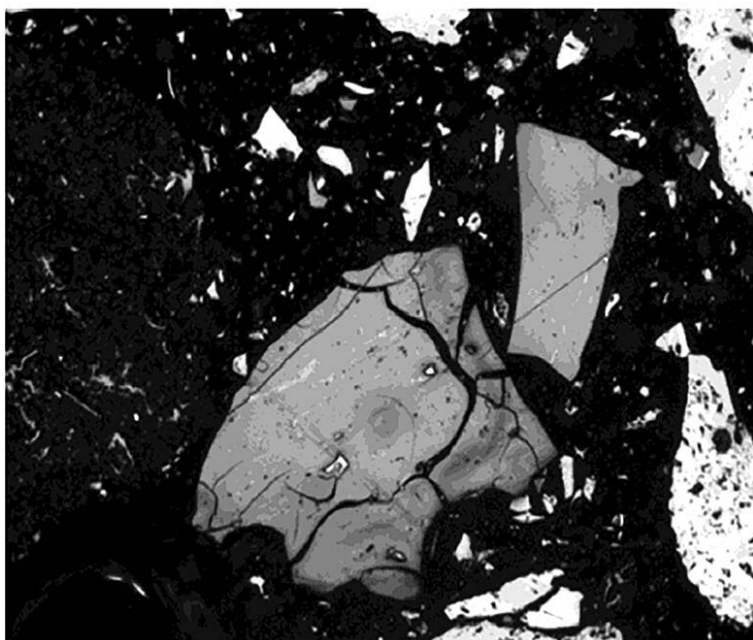
Рисунок А.6 — Клиновидные и разветвленные трещины
