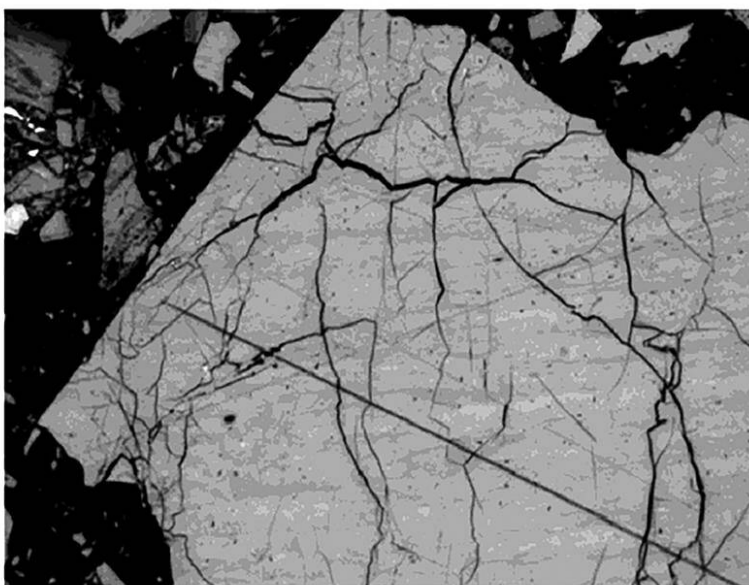
Рисунок А.8 — Клиновидные и разветвленные трещины, проникающие в глубину зерна
