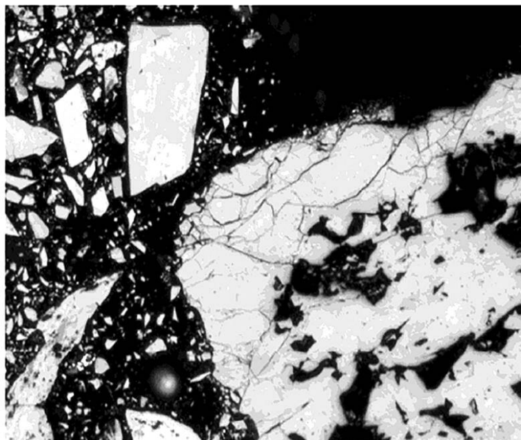
Рисунок А.13 — Дезинтеграция зерна угля с пустотами и многочисленными трещинами
