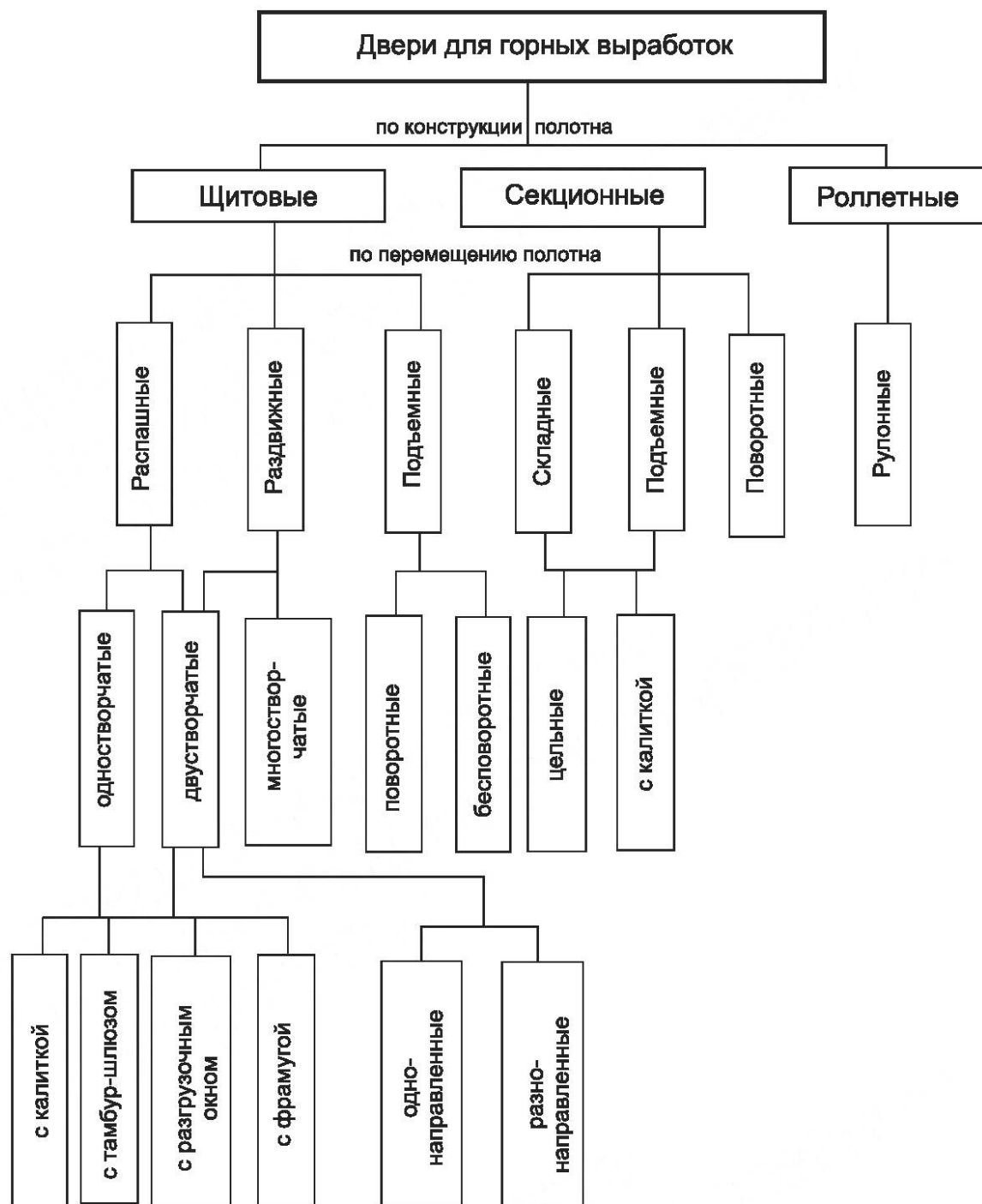
Рисунок 1 — Классификация дверей для горных выработок
