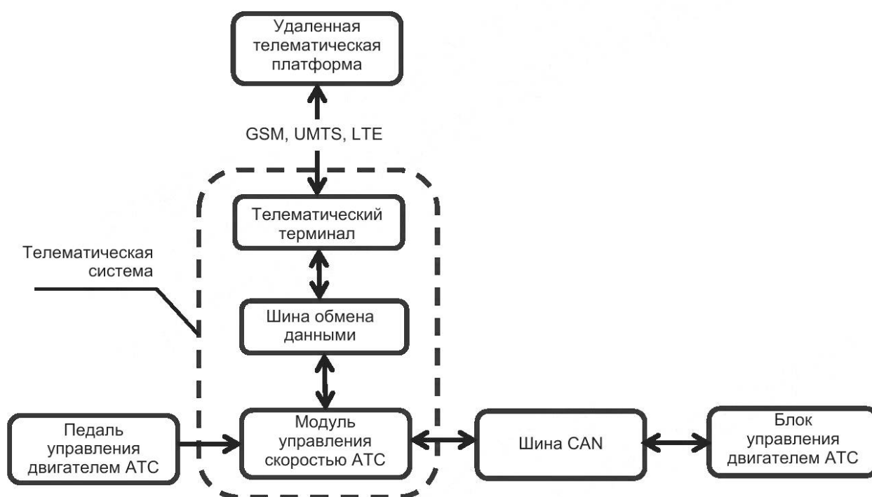
Рисунок 1 — Блок-схема телематической системы
