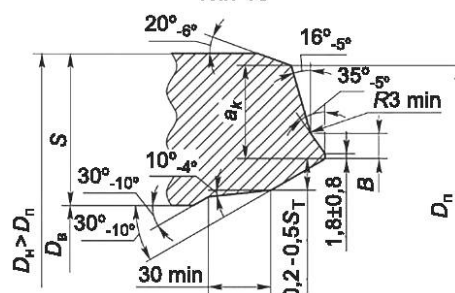
Для S_T > 15 мм, D_B < D_{BT} Тип 20
