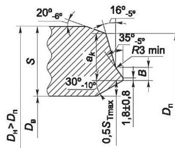
Для S_T > 15 мм, D_B < D_{BT}
