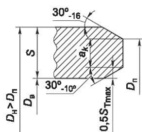
Для S_T \leq 5 мм, D_B < D_{BT} Тип 14
