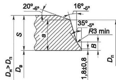
Для S_T > 15 мм, D_B = D_{BT} Тип 13
