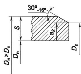
Для S_T \leq 5 мм, D_B = D_{BT} Тип 11
