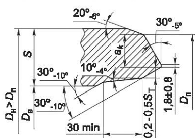
Для S_T \leq 15 мм, D_B < D_{BT} Тип 19
