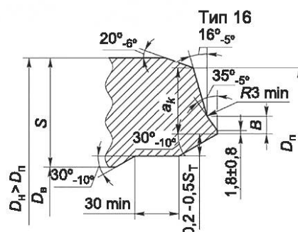
Для S_T > 15 мм, D_B < D_{BT} Тип 18
