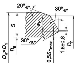
Для 5 \leq S_T \leq 15 мм, D_B = D_{BT} Тип 12
