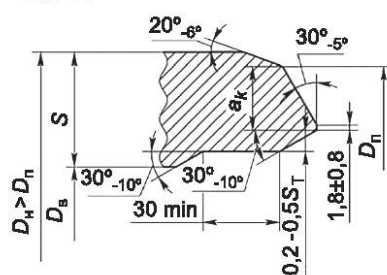
Для S_T \leq 5 мм, D_B < D_{BT} Тип 14
