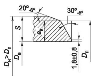
Для 5 \leq S_T \leq 15 мм, D_B = D_{BT} Тип 12
