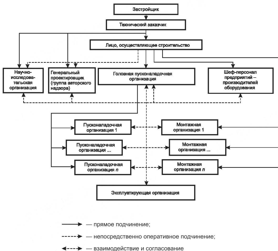
Рисунок А.1 — Типовая форма организационной структуры производства ПНР
