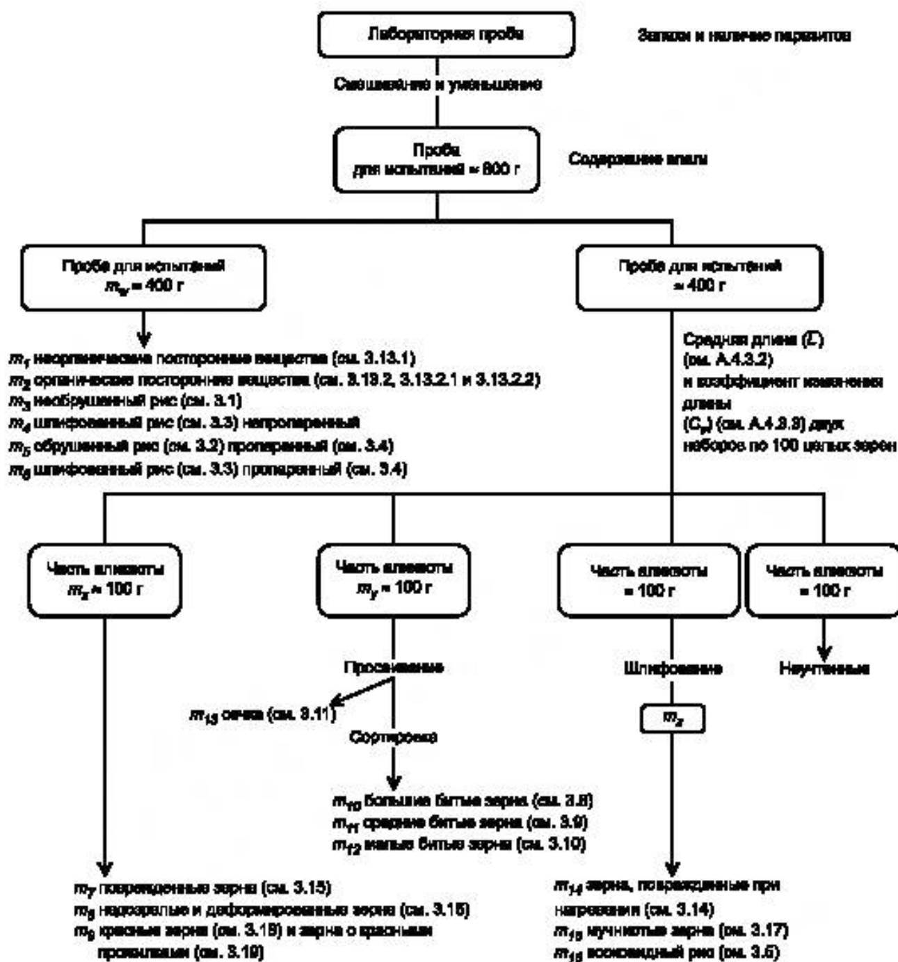
Рисунок A.1 — Схема определения категории зерна для обрубленного риса непропаренного
