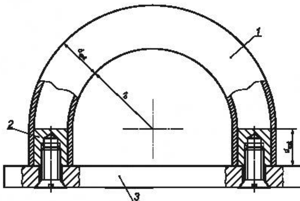
Рисунок 1 — Схема установки рукава для метода 1
