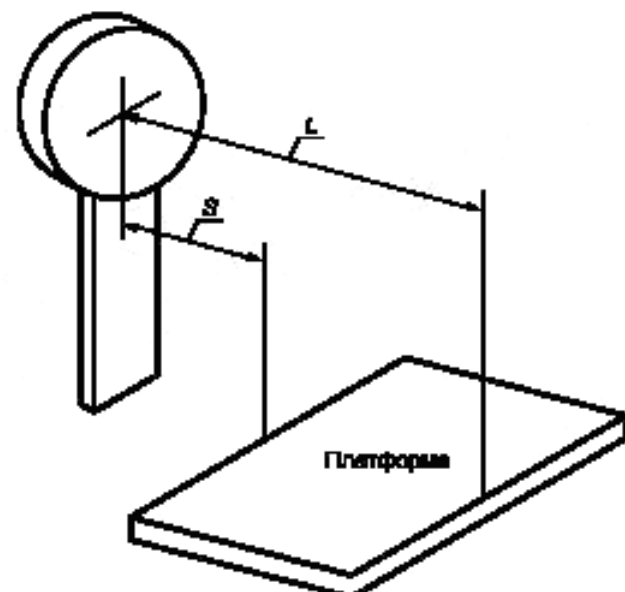
Рисунок 2 — Иллюстрация к термину «минимальное расстояние для снятия отсчета»
