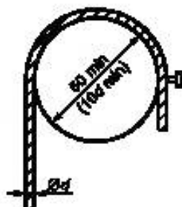
Рисунок 1 — Устройство для удерживания испытуемого образца корда
