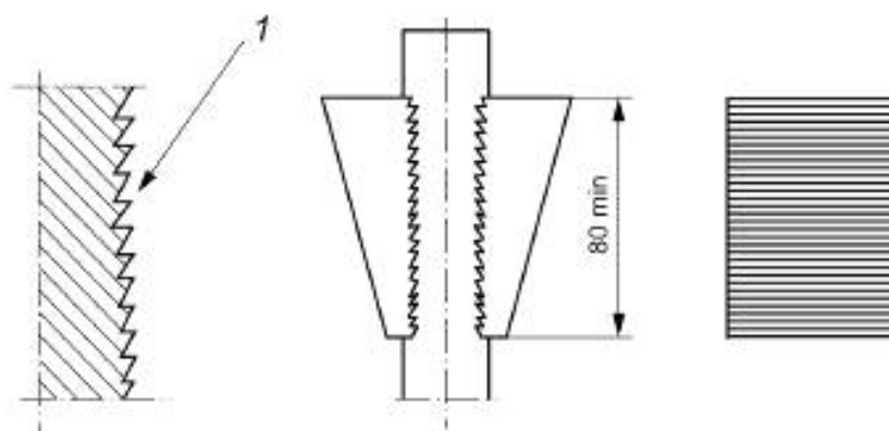
1 — детальное изображение ребер зажима
