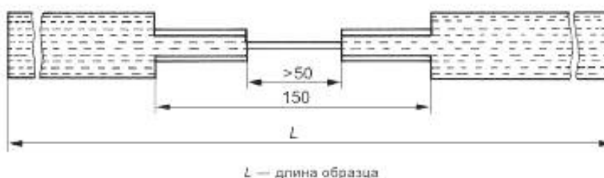
Рисунок 3 — Образец типа В
