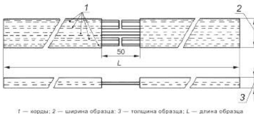
Рисунок 2 — Образец типа А
