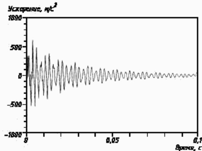
а) Сигнал ускорения после применения экспоненциального окна
