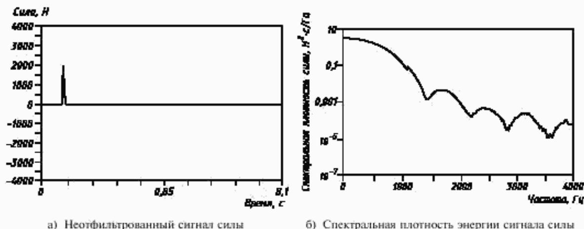
Рисунок 3 — Типичный импульс силы и его спектр
