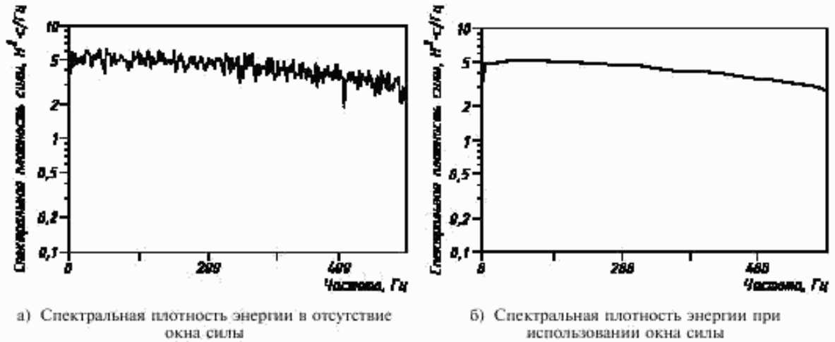
Рисунок 7 — Влияние окна силы на спектр сигнала силы
