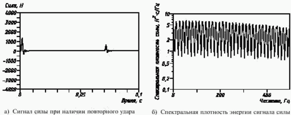
а) Сигнал силы при наличии повторного удара
