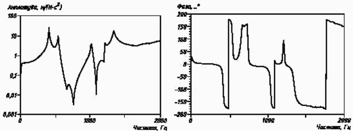
б) Ускоримость, полученная после применения окна
