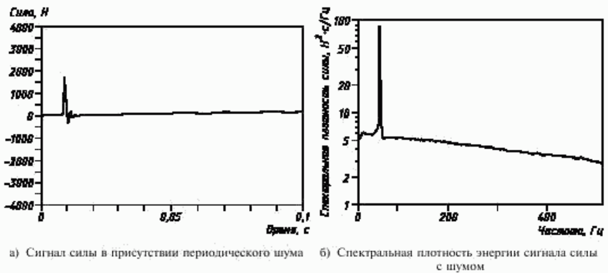
Рисунок 7 — Влияние окна силы на спектр сигнала силы
