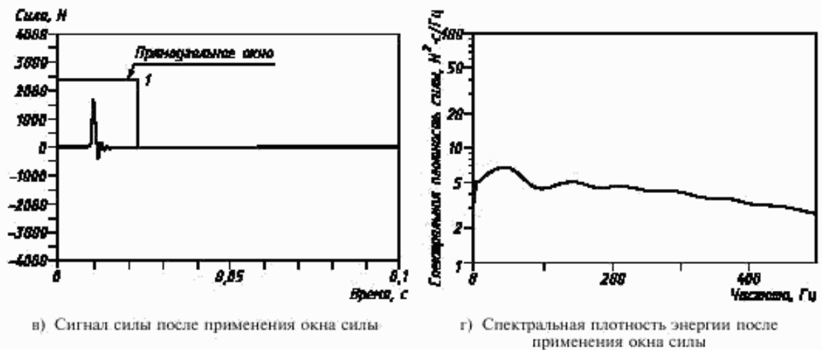
Рисунок 8 — «Просачивание», вызванное применением окна силы
