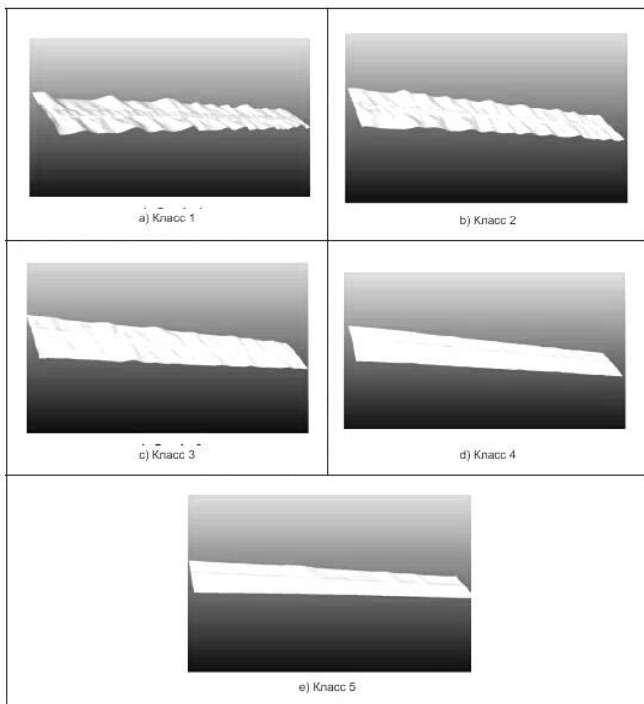
Рисунок А.10 — Измеренные изображения эталонов двойных швов
