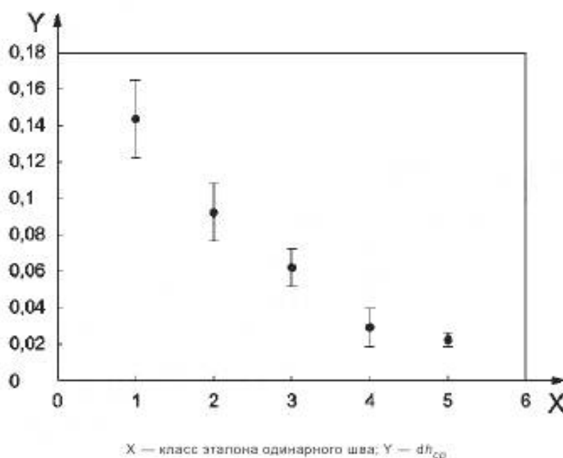
Рисунок А.7 — Соотношение между классом эталона одинарного шва и средним значением частоты высоты
