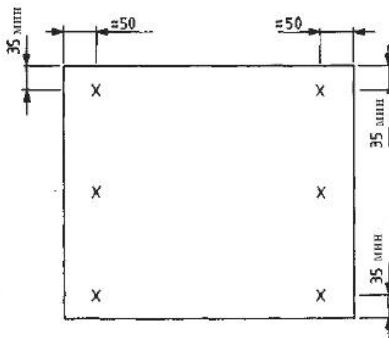
Рисунок 2 — Маркировка образцов для испытаний
