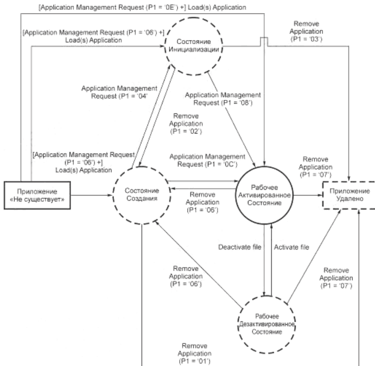
Рисунок 2 — Диаграмма жизненного цикла приложения
