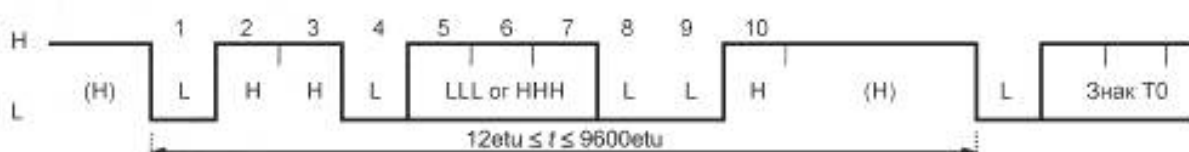
Рисунок 11 — Начальный знак TS
