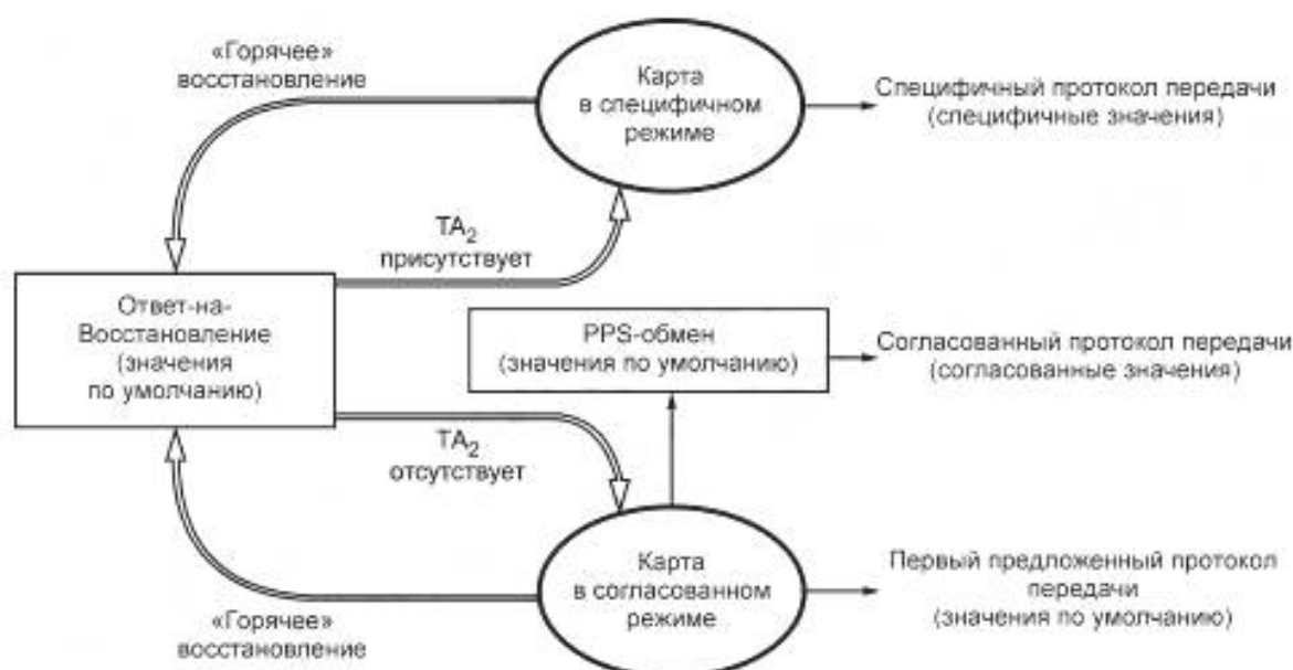
Рисунок 4 — Выбор параметров передачи и протокола
