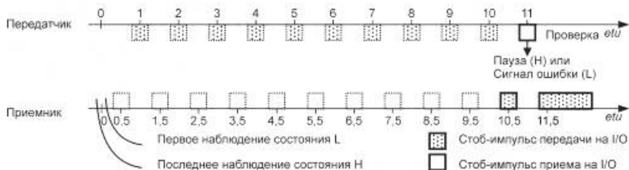
Рисунок 10 — Временные соотношения сигнала ошибки
