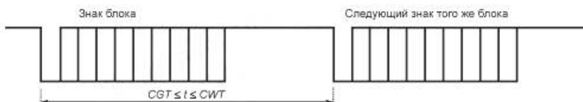
Рисунок 21 — Время ожидания знака в пределах блока
