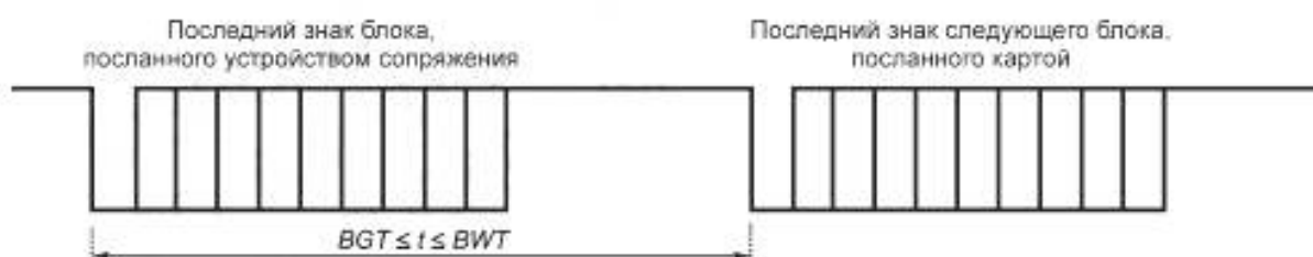
Рисунок 22 — Время ожидания блока
