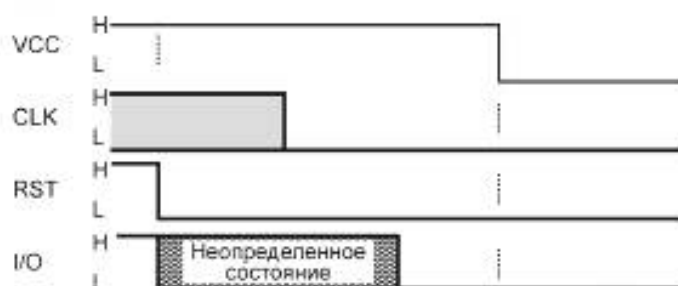
Рисунок 6 — Деактивация
