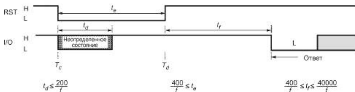
Рисунок 2 — «Горячее» восстановление
