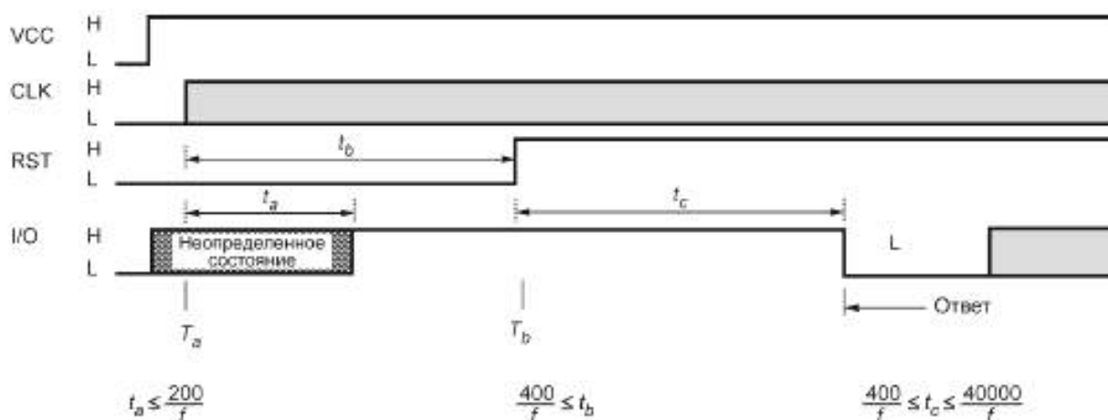
Рисунок 1 — Активация и «холодное» восстановление
