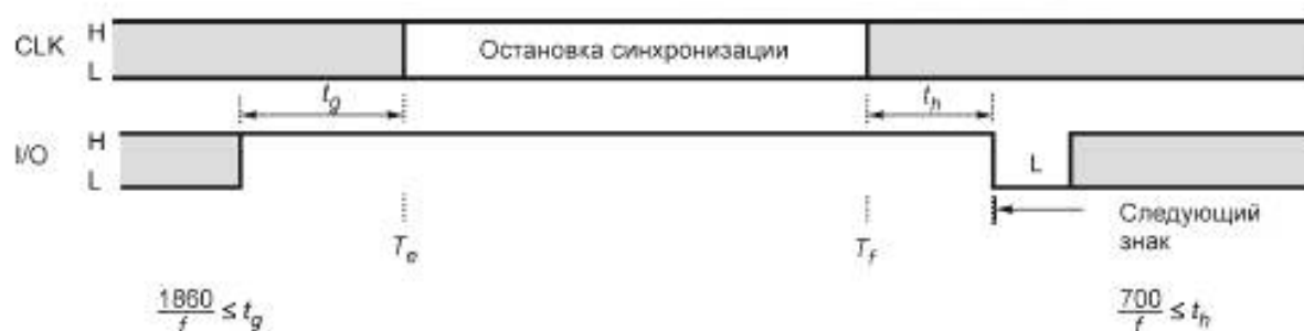
Рисунок 5 — Остановка синхронизации
