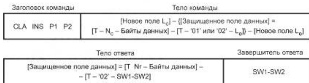
Рисунок 6 — Защищенная пара команда-ответ
