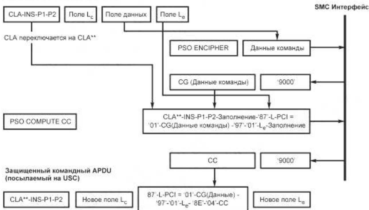
Рисунок B.1 — Создание защищенного командного APDU
