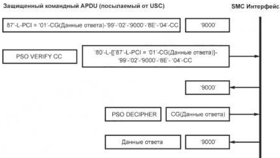
Рисунок В.2 — Создание защищенного ответного APDU
