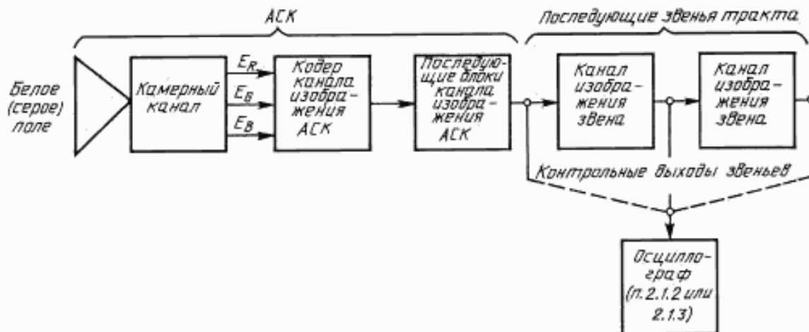
Структурная схема для измерения параметров сигнала гашения
