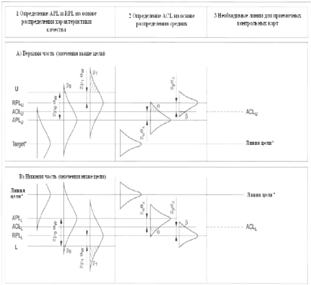
Рисунок 2 –Границы и определяющие элементы приемочных контрольных карт
