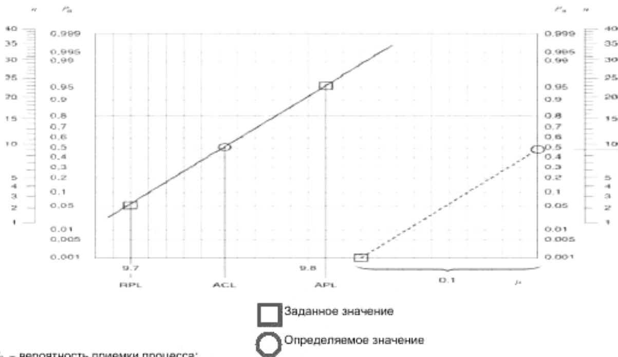
Рисунок А.2 –Построение приемочной контрольной карты. Односторонняя область допустимых значений
