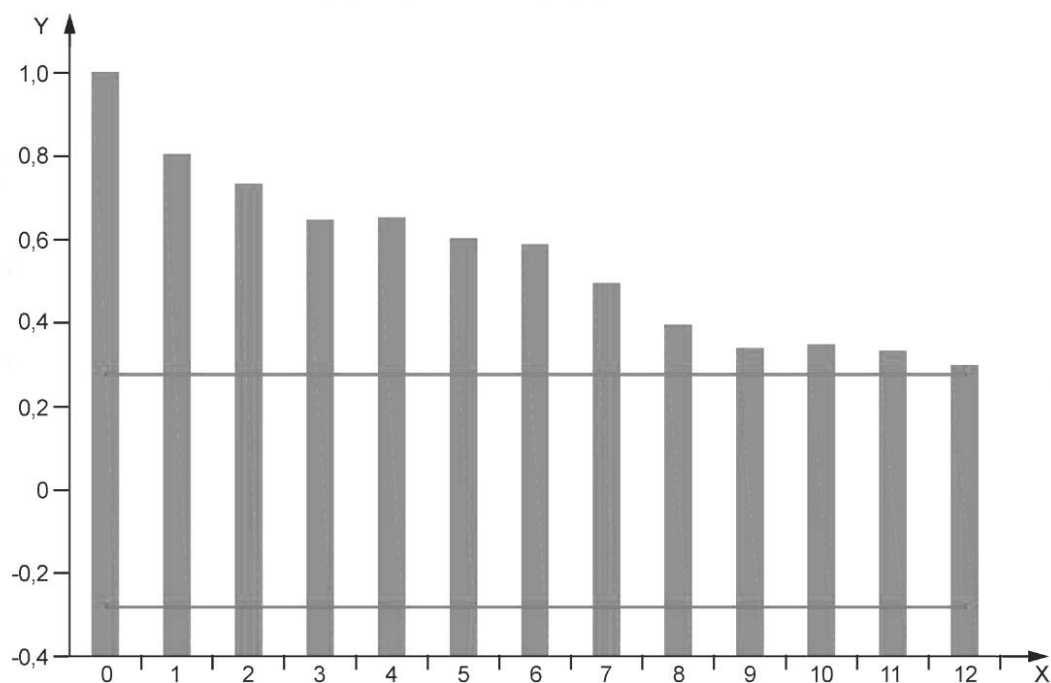
Рисунок 2 — Выборочные автокорреляции для серии ежедневных измерений вязкости и приближенный доверительный интервал с уровнем доверия 95 %
