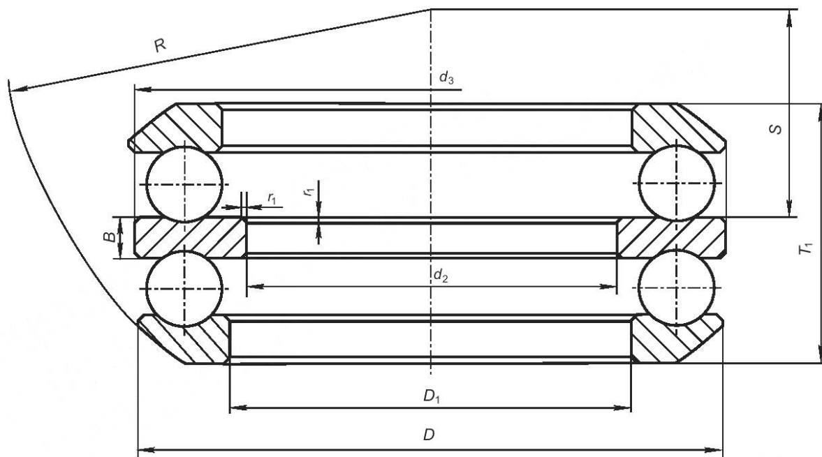
Рисунок 6 — Конструктивное исполнение 05
