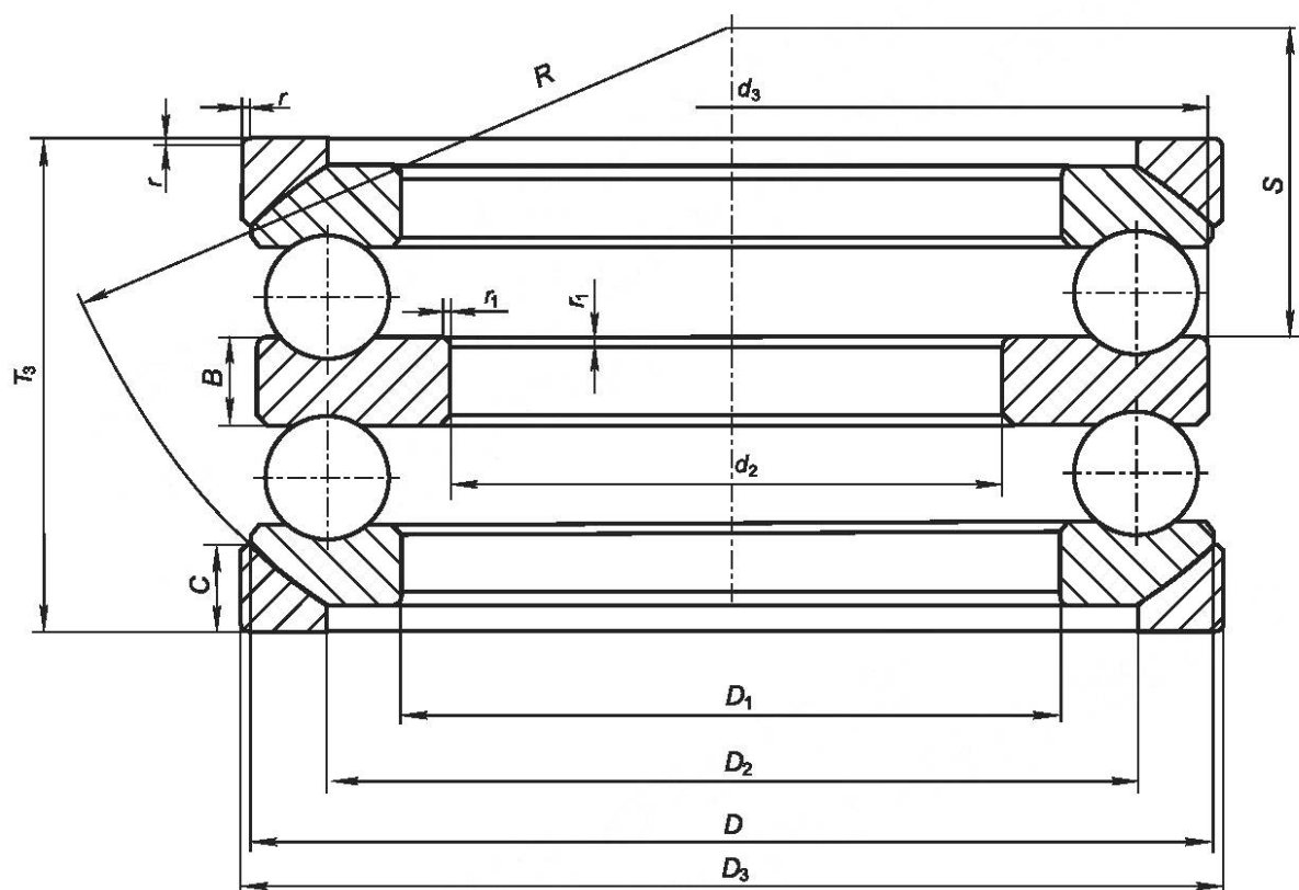
Рисунок 5 — Конструктивное исполнение 04
