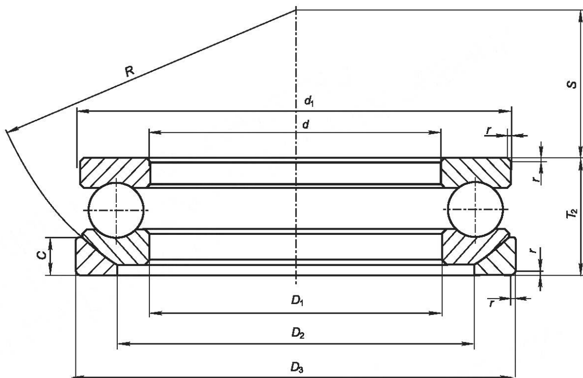
Рисунок 2 — Конструктивное исполнение 01
