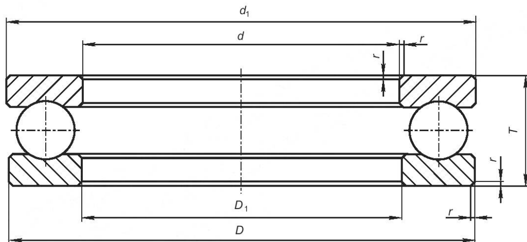
Рисунок 1 — Конструктивное исполнение 00
