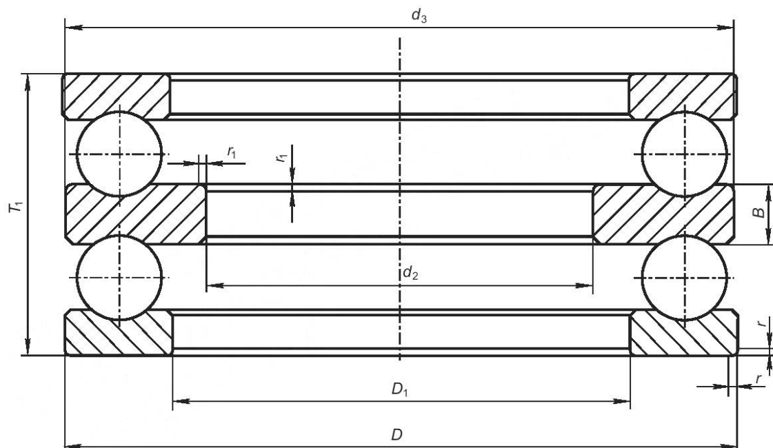
Рисунок 4 — Конструктивное исполнение 03
