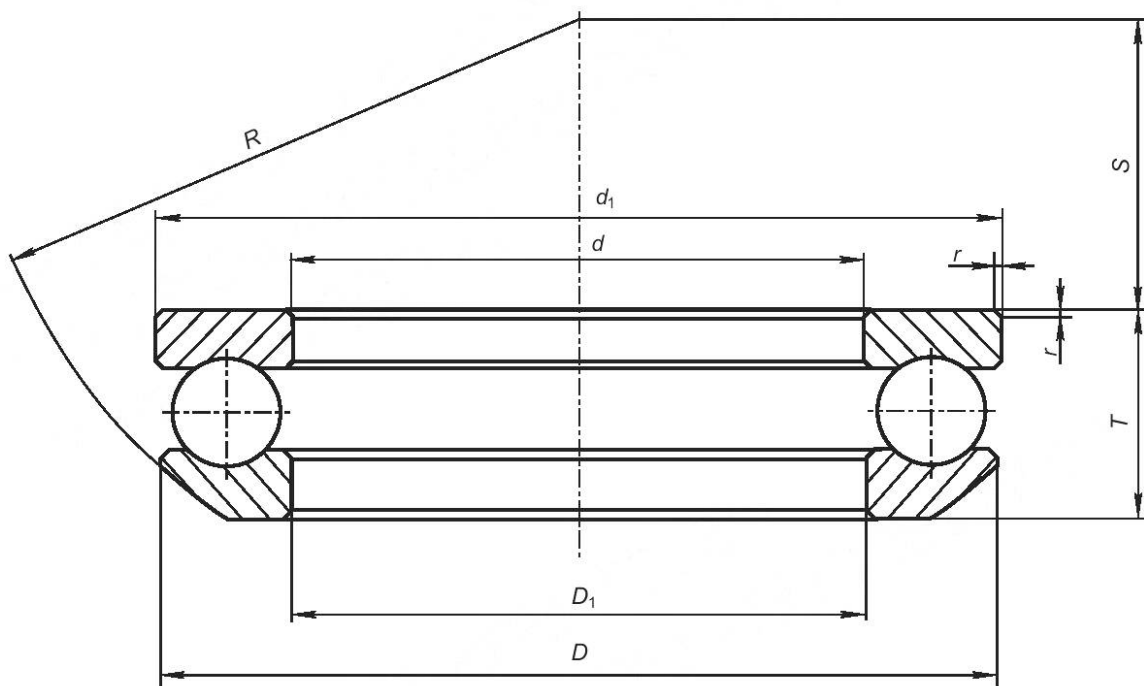
Рисунок 3 — Конструктивное исполнение 02
